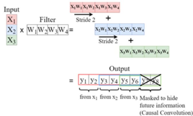
図2 転置畳み込みネットワーク
