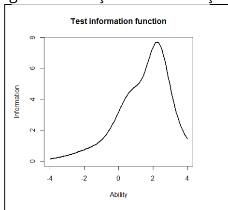
Figura 5 – Função de informação do teste
