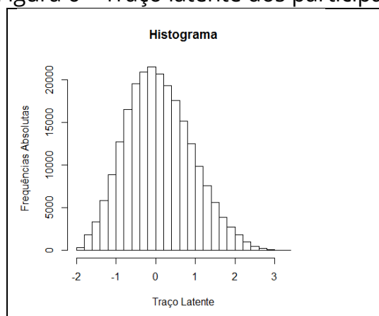
Figura 6 – Traço latente dos participantes
