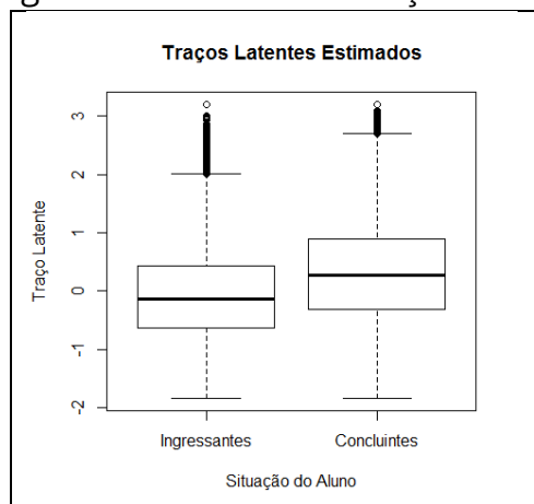
Figura 8 – Box-Plot do traço latente
