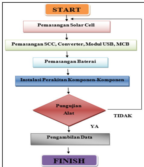
Gambar 1. Flowchart pemasangan alat pada station charger handphone
