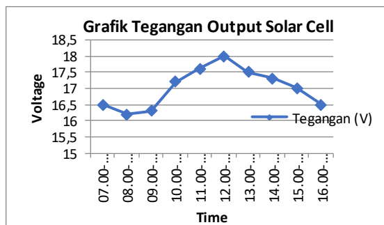
Gambar 3. Grafik Tegangan Output Solar cell
