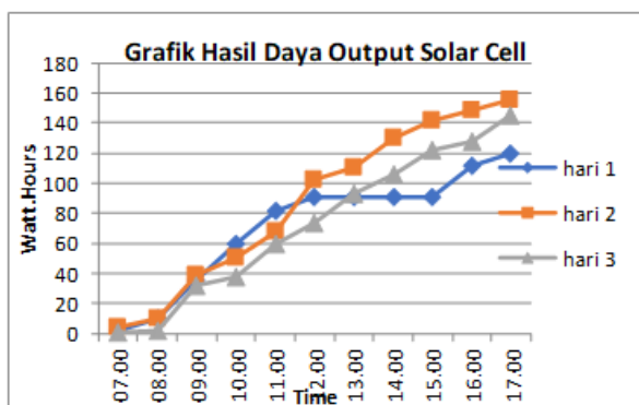
Gambar 4. Grafik Hasil Daya Output Solar cell
