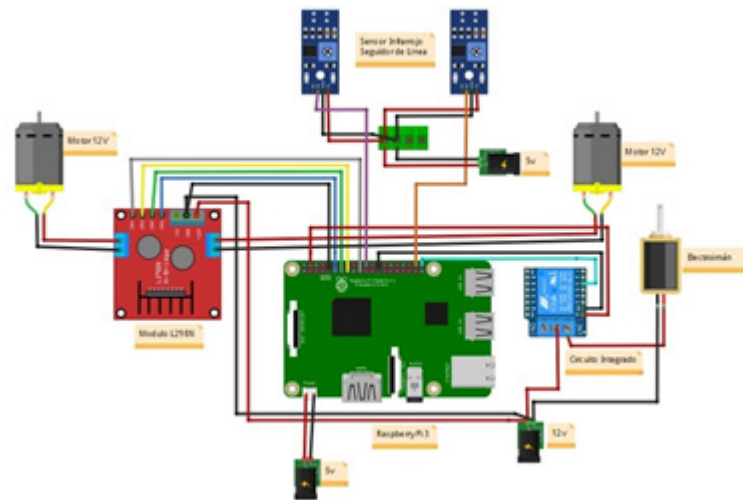
Figura 4. Integración de componentes eléctricos-electrónicos Fuente: elaboración propia
