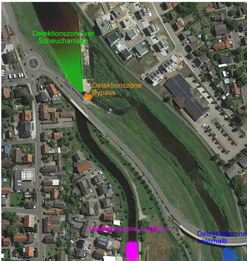
Abb. 180: Detektionszonen in Rotenfels zur Aufnahme der Signale der besenderten Aale während der Versuchsdurchführung vom 09.11.2016 bis 04.03.2017.
