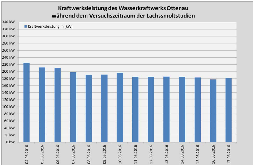
Abb. 129: Kraftwerksleistung im Versuchszeitraum vom 04.05.-17.05.2016 mit nur leicht schwankenden Abflüssen in Richtung des Wasserkraftwerks im Kraftwerkskanal und damit auch vor dem Schrägwehrechen.
