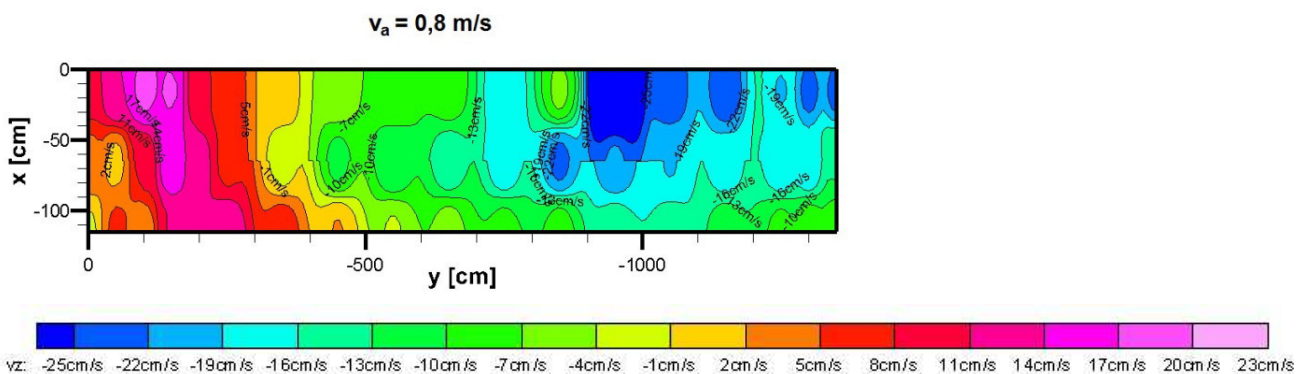
Abb. 77: Strömungsdiagramm mit Darstellung der z-Komponente der Strömungsgeschwindigkeit des Schrägrehens Ottenau im Schnitt 5 ( z = -1,30 \text{ m} ) und mit einer Anströmgeschwindigkeit von 0,8 \text{ m/s} (Quelle: verändert nach Schwab, 2016).
