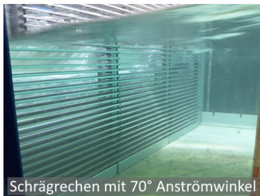
Abb. 95: Verschiedene Anströmwinkel mittels modularem Rechensystem im Forschungslabor der TU Darmstadt.
