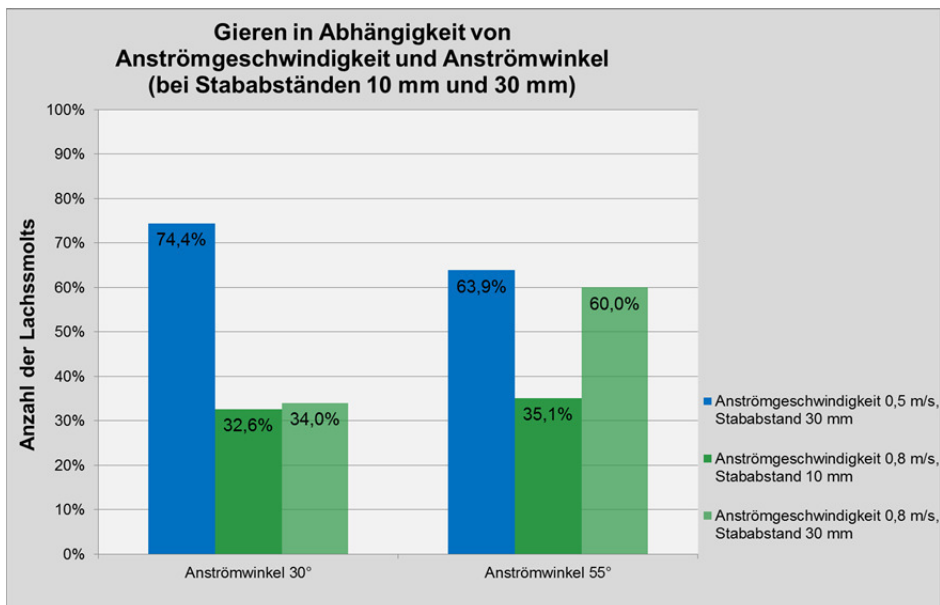
Abb. 113: Häufigkeit des Gierens bei Stababständen von 10 mm und 30 mm in Abhängigkeit von Anströmgeschwindigkeit und Anströmwinkel.
