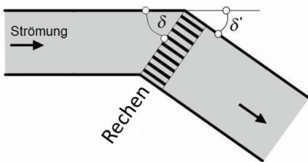
Abb. 28: Definition des Anströmwinkels \delta und des Komplementärwinkels \delta' nach Meusburger ( Quelle: Meusburger, 2002; verändert von Glock 2017 ).
