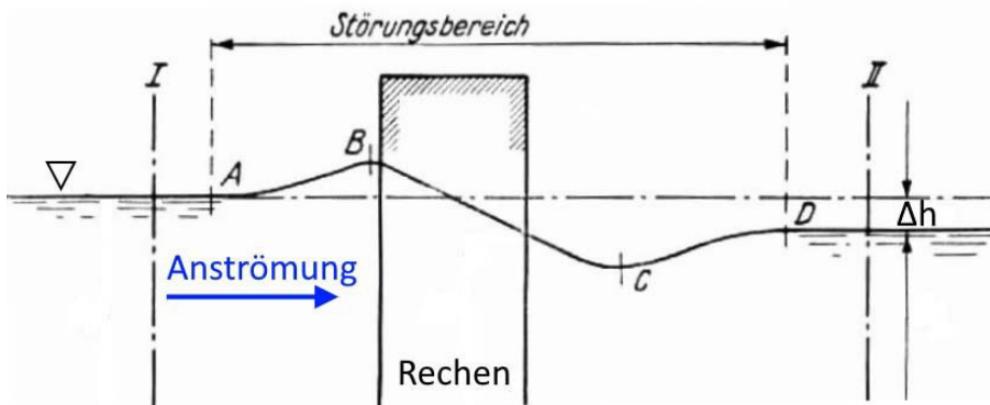
Abb. 10: Wasserspiegellinie im Störungsbereich eines Rechens mit dem Wasserspiegelunterschied \Delta h ober- und unterwasserseitig des Rechens (Quelle: verändert nach Kirschmer, 1925).
