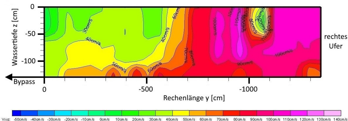
Abb. 72: Tiefendiagramme der Strömungsfelder parallel zur Rechenebene, a) bei einer Anströmgeschwindigkeit von 0,4 m/s und b) bei 0,5 m/s mit Blick in Fließrichtung/Unterwasser (Quelle: verändert nach Schwab, 2016).
