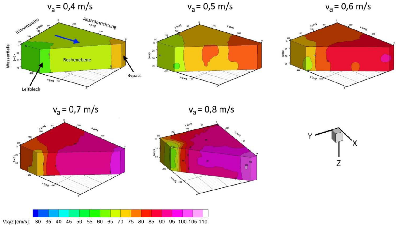
Abb. 107: Strömungssignaturen bei Anströmgeschwindigkeiten von 0,4 bis 0,8 m/s mit Zunahme von Geschwindigkeiten und Inhomogenitäten. Die Stababstände betragen 18 mm, der Anströmwinkel 45^\circ (Quelle: verändert nach Schwab, 2016).
