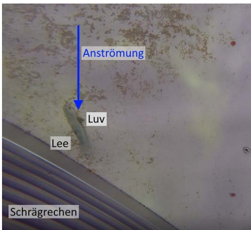
Abb. 13: Lachssmolt vor einem Schrägrechen, auf dessen Luvseite Überdrücke wirken und auf seine Leeseite Unterdrücke.
