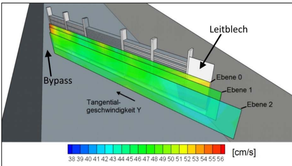
Abb. 101: Tangentiale Geschwindigkeitskomponente an der rechten Rinnenwand erhöht aufgrund Leitblech bei Anström winkel von 30°, Stababstand von 18mm und Anströmgeschwindigkeit von 0,5 m/s (Quelle: verändert nach Glock, 2017).
