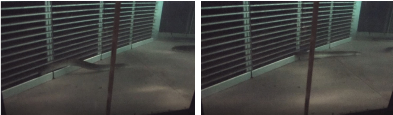
Abb. 149: Stromaufwärts gerichtetes Suchverhalten eines Aals bei Versuch-Nr. V15.1, welcher die Rechenebene entlang schwamm, den Schrägrechen mehrfach berührte (links) und anschließend ab ca. Rechenmitte Richtung Oberstrom schwamm (rechts).
