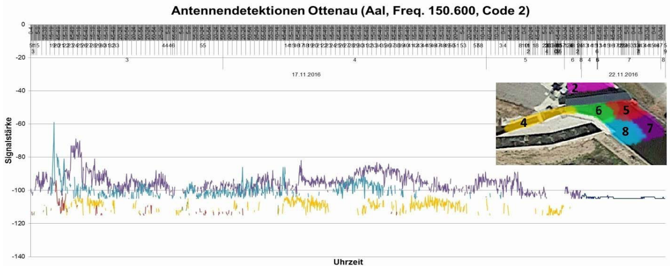
Abb. 170: Signalstärken, welche das Verhalten des Aals mit Code-Nr. 2 am 17.11.2016 zwischen 3 Uhr und 8 Uhr vor dem Schrägrechen und in der Ausleitungsstrecke Ottenau wiedergeben.
