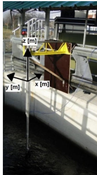
Abb. 69: Links Querschnitt des Schrägwehres Ottenau mit Messebenen auf der x-Achse sowie der z-Achse in die Tiefe (Quelle: verändert nach Schwab, 2016). Rechts Foto des Messwagens mit Messgerät samt Koordinatensystem (Quelle: Schwab, 2016).
