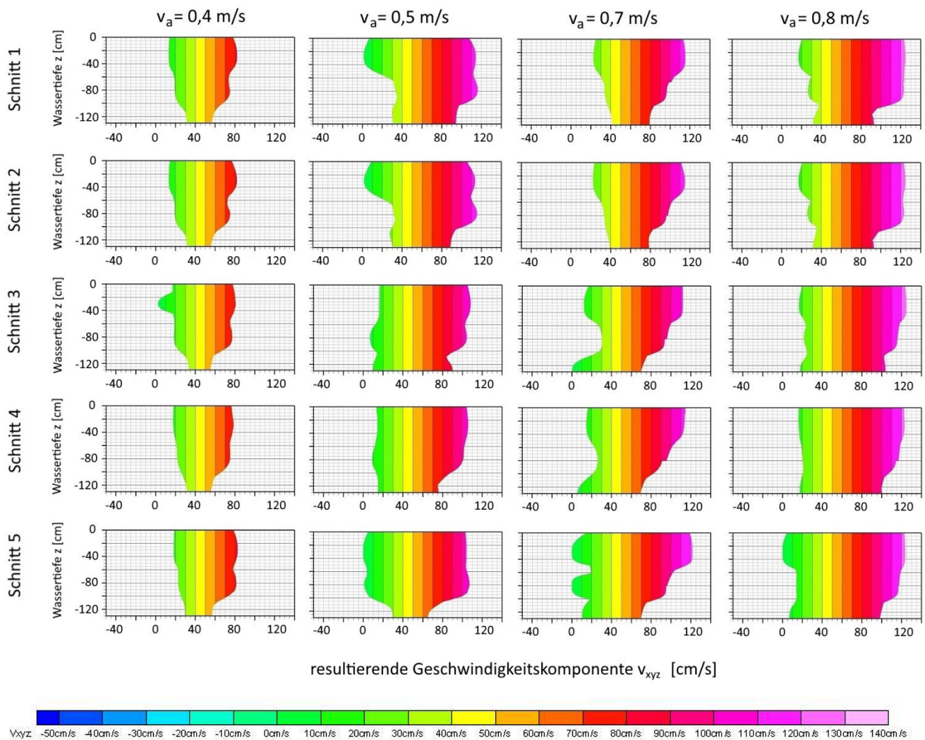
Abb. 70: Geschwindigkeitsprofile aller fünf Ebenen der x-Achse (Tab. 18) und aller eingestellten Anströmgeschwindigkeiten. Die Profilbilder sind über die Wassertiefe z aufgetragen und stellen den gesamten Messquerschnitt der gemessenen resultierenden Geschwindigkeitskomponente v_{xyz} für jede Anströmgeschwindigkeit und jeden Tiefenschnitt dar (Quelle: verändert nach Schwab, 2016).
