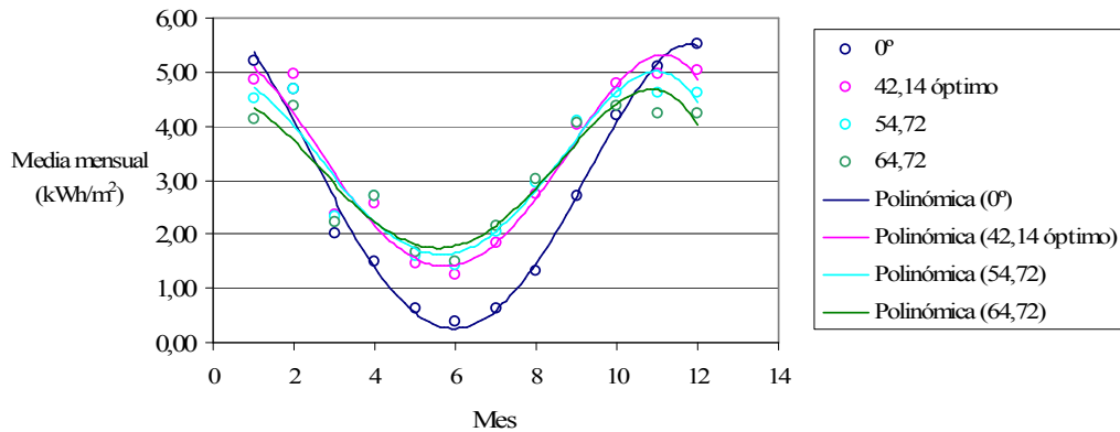
Figura 5: Variación mensual de la energía solar media diaria colectada por un plano inclinado los ángulos que se indican en la estación Ushuaia.
