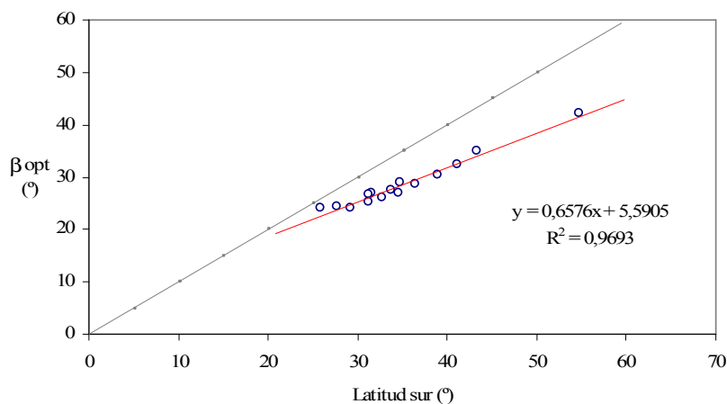
Figura 2: Variación del ángulo óptimo con la latitud para las estaciones consideradas en el trabajo (excluyendo a Almirante. Brown); se incluye la recta que corresponde al ángulo óptimo igual a la latitud.
