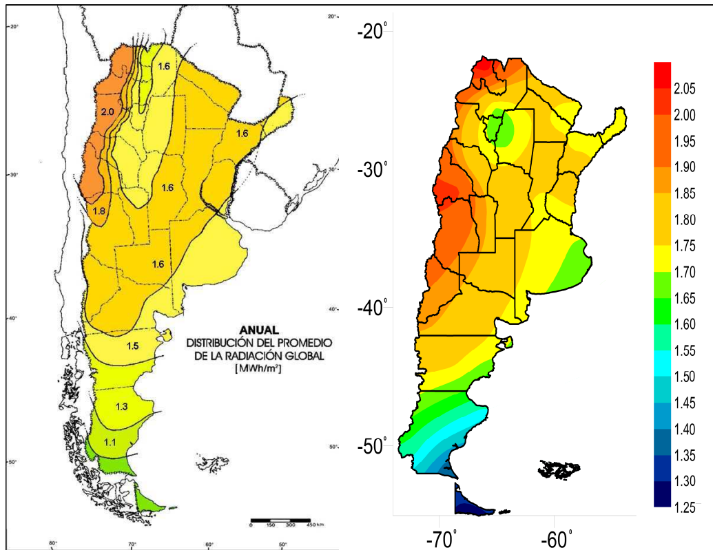
Figura 1: (Izquierda) Distribución del promedio anual acumulado de la radiación global sobre plano horizontal (adaptado de Grossi Gallegos, 1998) y (derecha) sobre planos inclinados un ángulo óptimo (Righini y Grossi Gallegos, 2011); la unidad de la escala es MWh/m^2 .
