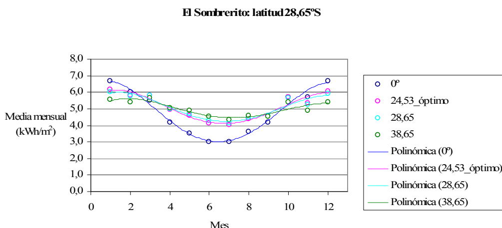
Figura 4: Variación mensual de la energía solar media diaria colectada por un plano inclinado los ángulos que se indican en la estación El Sombrerito.
