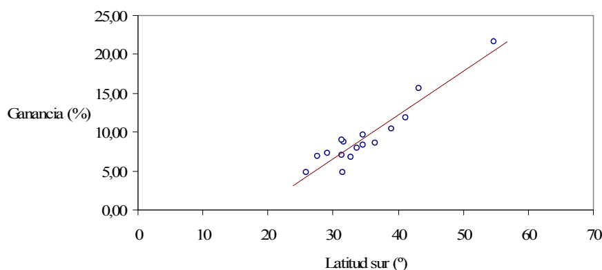
Figura 3: Ganancia relativa porcentual con respecto al plano horizontal obtenida al inclinar el plano el ángulo que optimiza la energía anual en función de la latitud del lugar.
