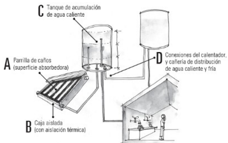
Banco de ensayos del calefón solar y esquema de sus componentes.
