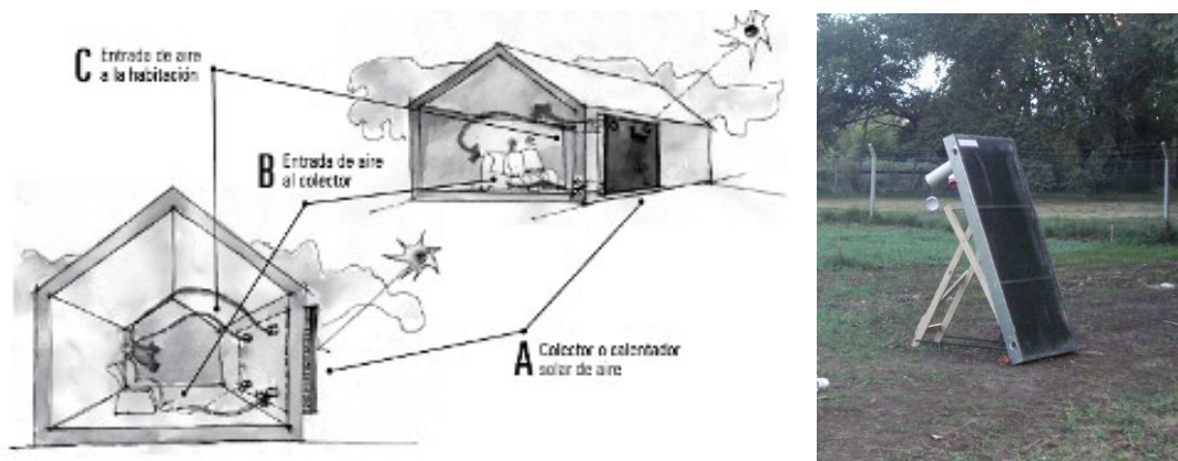
Esquema de funcionamiento del calentador de aire e imagen del mismo
