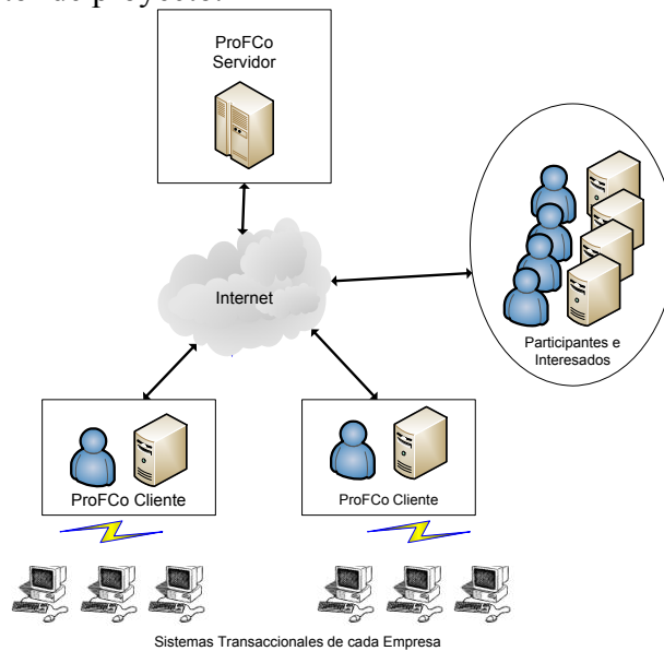
Figura 4. Arquitectura ProFCo
