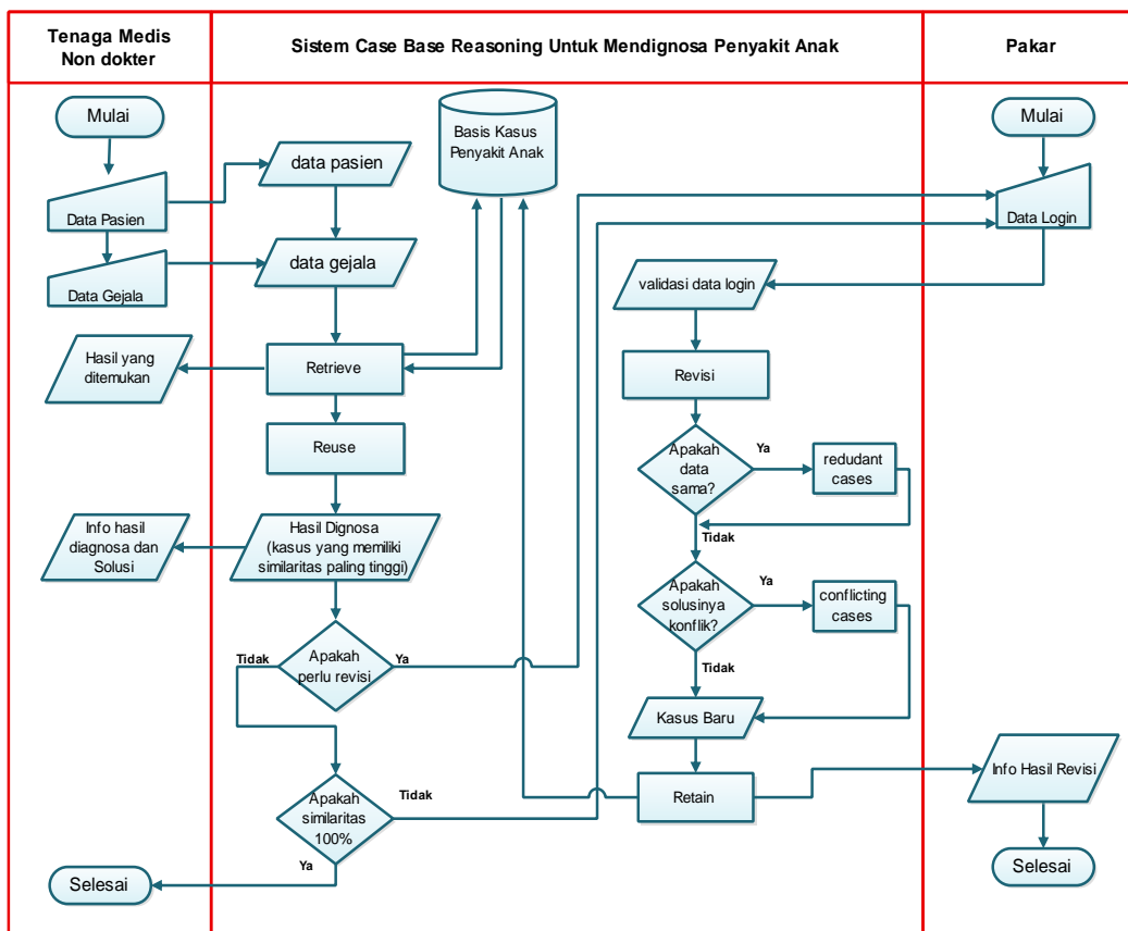
Gambar 2.1 Flowchart sistem CBR diagnosa penyakit anak
