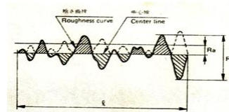
Gambar 4 : Profil Kurva Kekasaran
