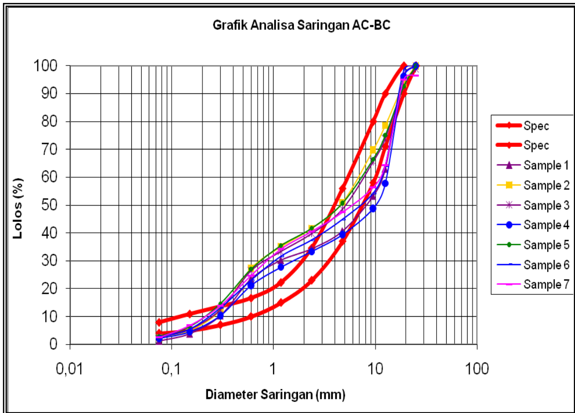
Gambar 6. Grafik Hasil Pengujian Analisa Saringan Sumber: Hasil Pengujian
