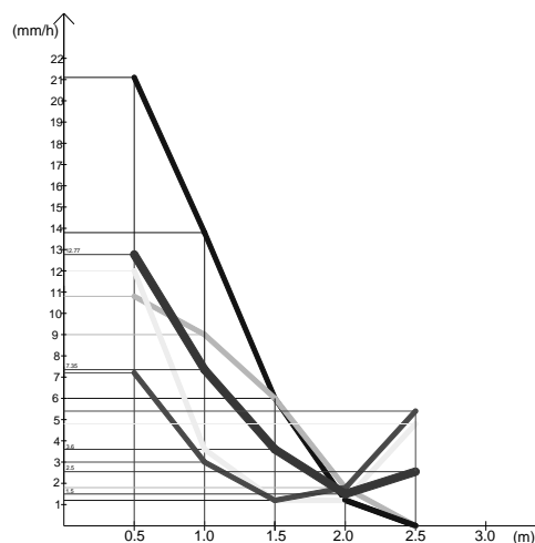
Graf. 3. Raspored vodenog taloga za Agridor 4190, Q = 20 \text{ l/h} , p = 2.5 \text{ bar}
