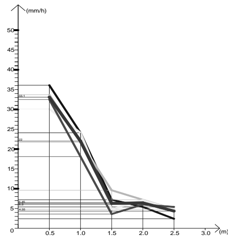
Graf. 7. Raspored vodenog taloga za Agridor 4190, za Q = 90 l/h, p = 2.5 bar
