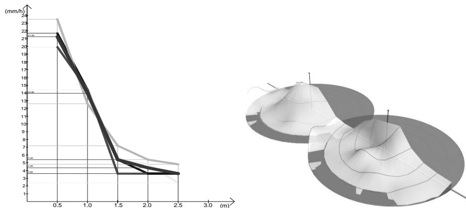
Graf. 6. Raspored vodenog taloga za Agridor 4190, za Q = 90 l/h, p = 2 bar
