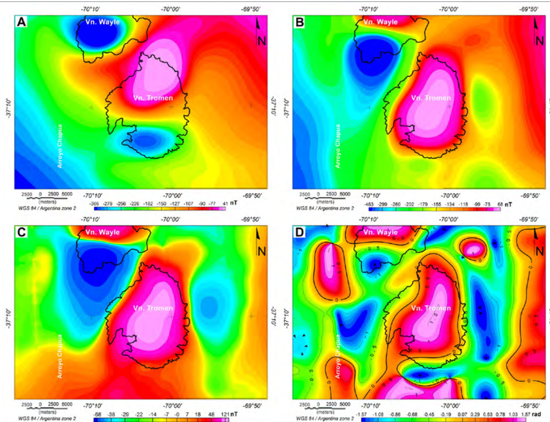
Figura 3. Mapas obtenidos del procesamiento de los datos aeromagnéticos en la zona del volcán Tromen. a) Anomalía magnética; b) Reducción al polo de las anomalías magnéticas; c) Anomalía residual obtenida al aplicar un filtro Butterworth de orden 8 y una longitud de onda de 40 km; d) Ángulo de Tilt aplicado a las anomalías magnéticas reducidas al polo, donde el contorno de valor cero indica los límites de las estructuras geológicas. En línea negra se representa la geometría de los volcanes Tromen y Wayle.
