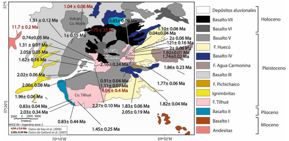
Figura 2. Mapa de las rocas volcánicas neógenas a holocenas del plateau del Tromen. Modificado de Galland et al. (2007).
