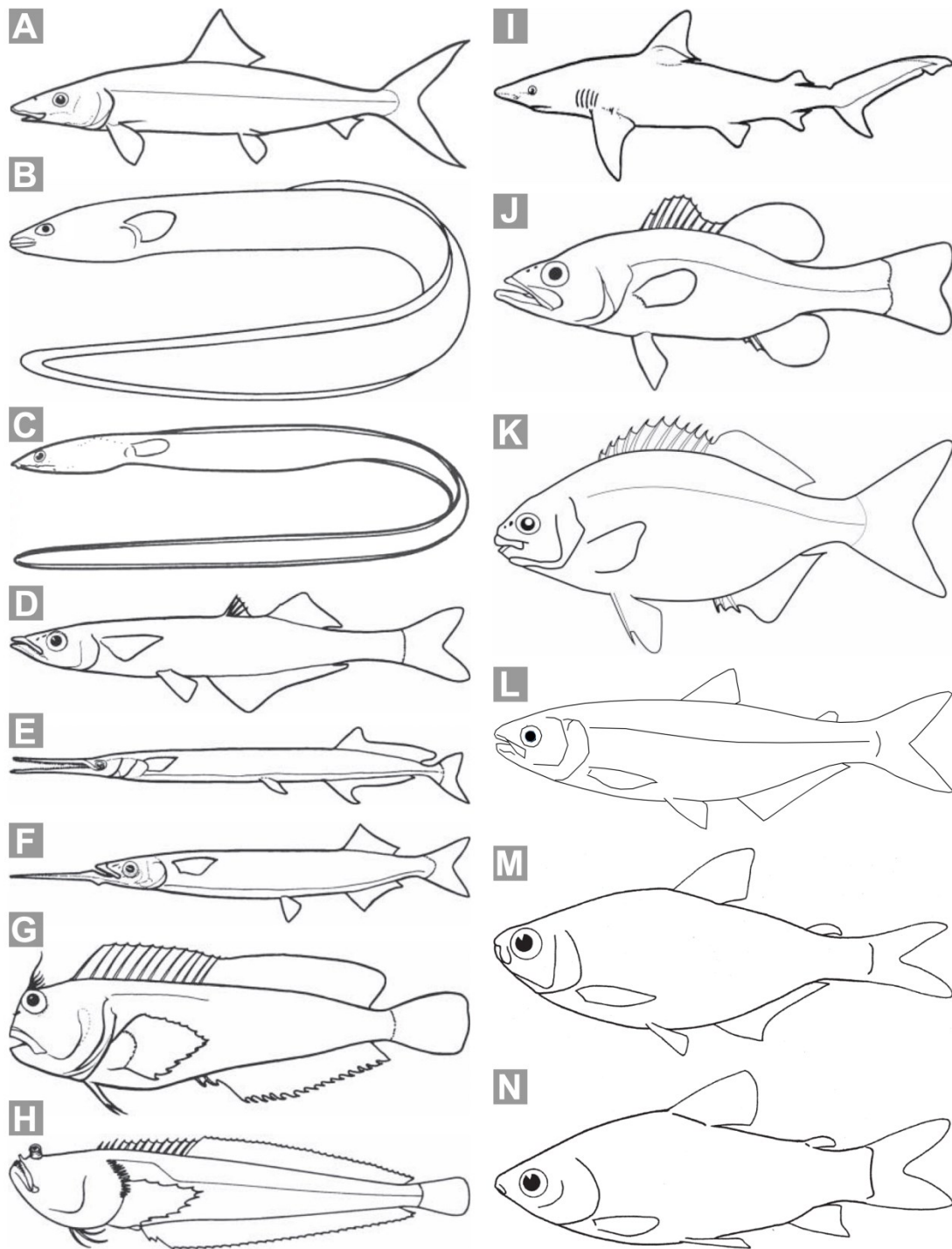
Fig. 1. Morfología externa generalizada/ilustrativa de un miembro de las familias Albulidae (A), Anguillidae (B), Ophichthidae (C), Atherinopsidae (D), Belontiidae (E), Hemiramphidae (F), Blenniidae (G), Dactyloscopidae (H), Carcharhinidae (I), Centrarchidae (J), Kyphosidae (K), Bryconidae (L), Characidae (M) y Curimatidae (N). Modificado de Nelson et al. (2016); L: Ilustración inédita.
