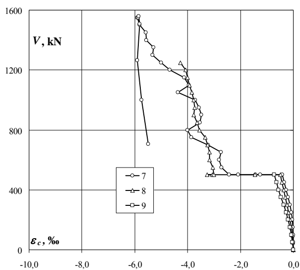
Beton – odkształcenia po stronie S i N (na słupie) ( \epsilon_c ) / Concrete – strains on S and N side (on the column) ( \epsilon_c )
