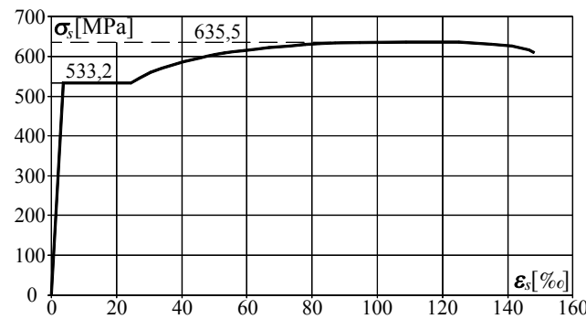
prętów zbrojeniowych Ø20 / reinforcement bars Ø20
