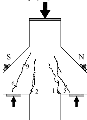
Układ rys przy sile 2000kN / Crack pattern at 2000kN
