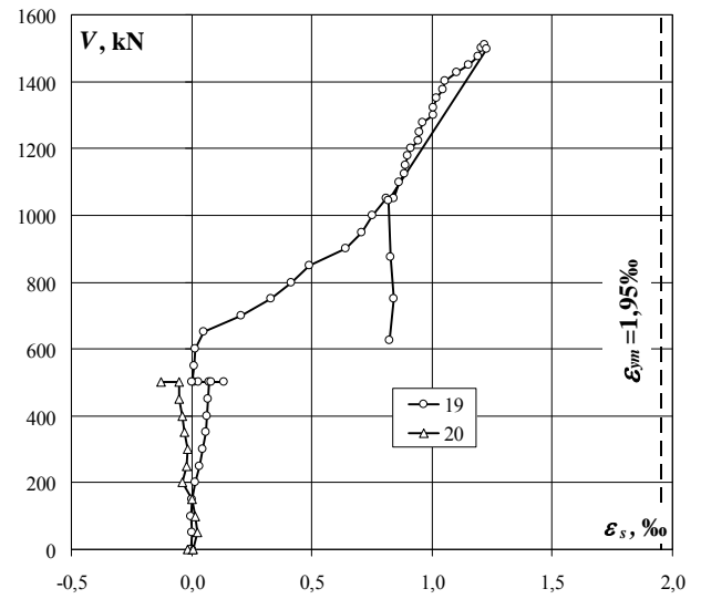
Strzemię 3 – odkształcenia po stronie S i N ( \varepsilon_s ) / Stirrup 3 – strains on S and N side ( \varepsilon_s )
