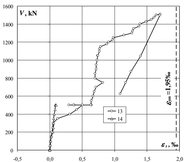
Strzemię 2 – odkształcenia po stronie S i N ( \varepsilon_s ) / Stirrup 2 – strains on S and N side ( \varepsilon_s )
