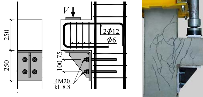
Rys. 3.25. Konstrukcja elementu C-III (szczegóły patrz załącznik) i widok zarysowania przy sile 477 kN Fig. 3.25. Design of element C – III (see annex for details) and crack pattern by force 477 kN
