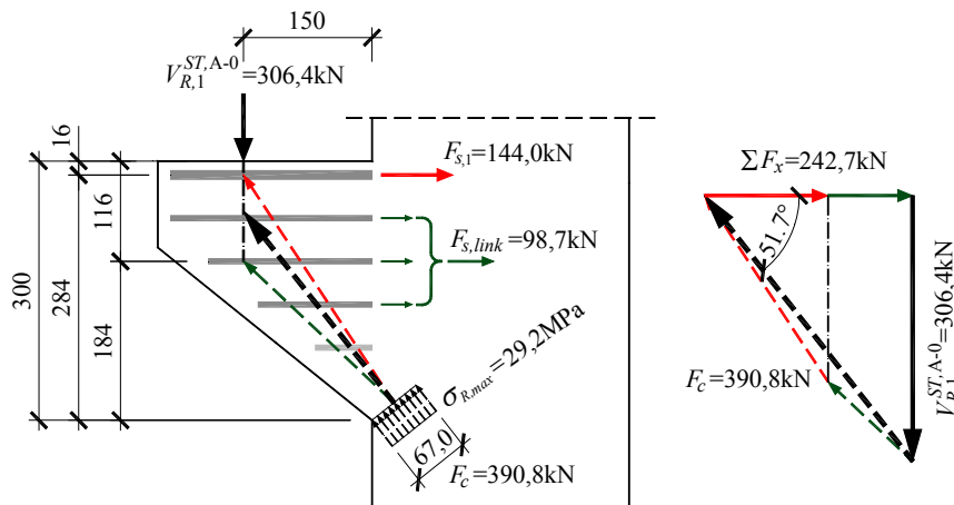
Rys. 3.15. Analiza nośności wspornika A – 0 za pomocą zmodyfikowanego modelu S-T
