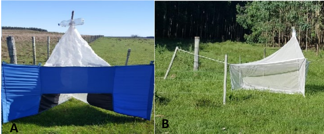
Figura 1. Trampas utilizadas para realizar capturas de tábanos. (A) Trampa Nzi y (B) trampa Malaise.
