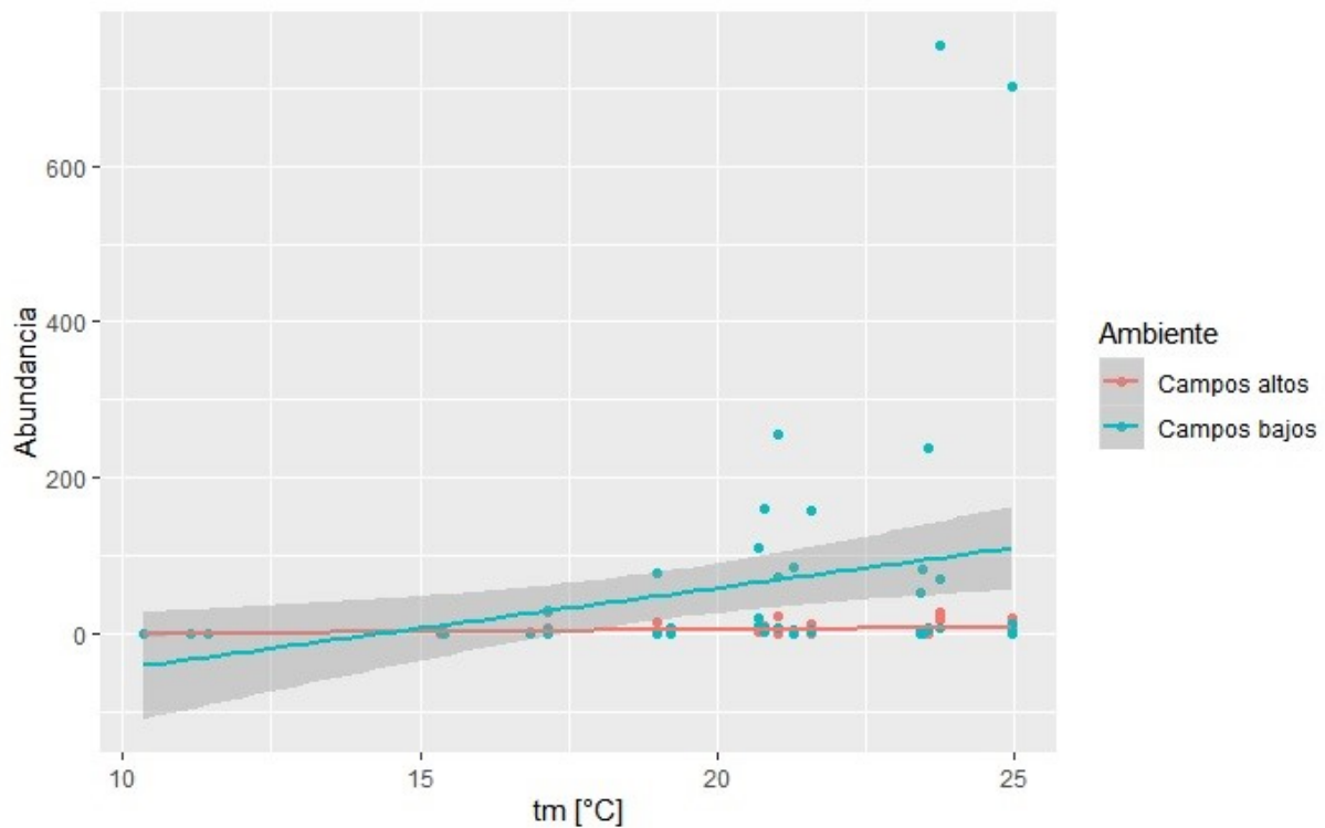
Figura 6. Abundancia de tábanos en Tacuarembó, Uruguay, en función de la temperatura media (° C) (tm), mes y año según el análisis GLM con una distribución cuasi-Poisson. Los modelos para cada ambiente son: Abundancia_{Campos\ altos} = \exp^{-6.886 + 0.386 * tm} y Abundancia_{Campos\ bajos} = \exp^{-4.391 + 0.386 * tm}
