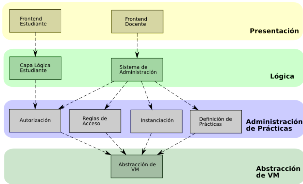
Figura 1. Arquitectura del Framework
