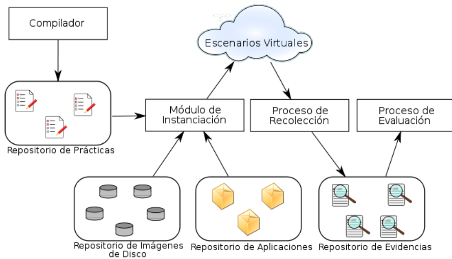
Figura 4. Componentes de la herramienta
