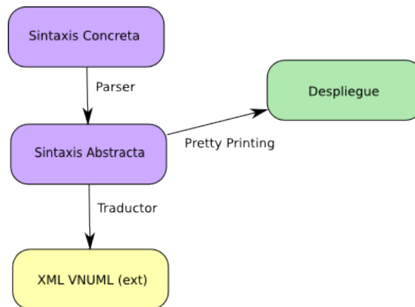
Figura 5. Módulos Involucrados en el Diseño del Compilador
