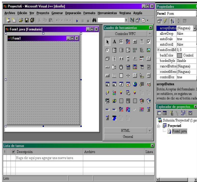
Figura 3.43 Entorno de desarrollo de Visual J++ 6.0
