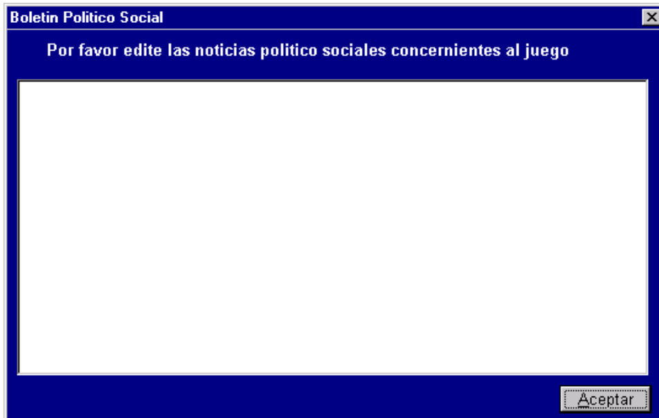
Figura 6.24. Boletín Político-Social
