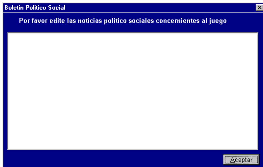
Figura 3.20 Noticias Político-Sociales
