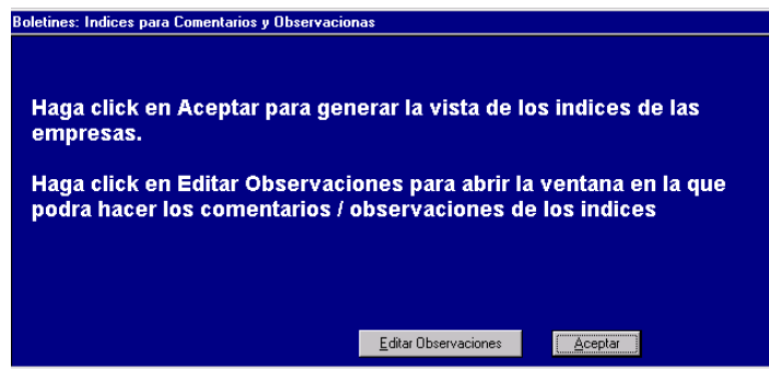
Figura 3.27 Mensajes
