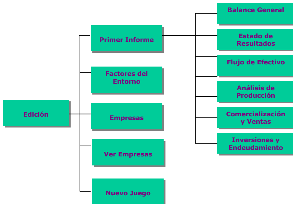
Figura 3.36 Modulo edición
