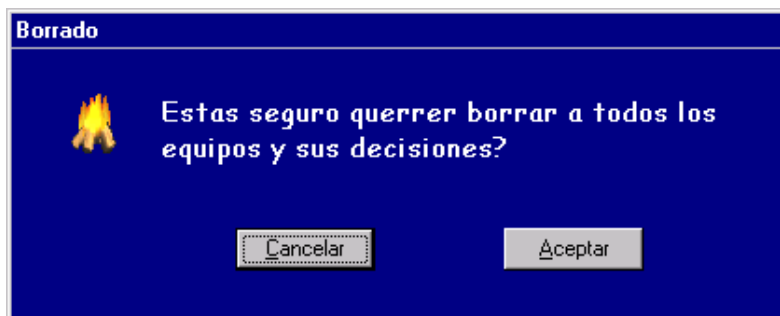
Figura 3.28 Alertas
