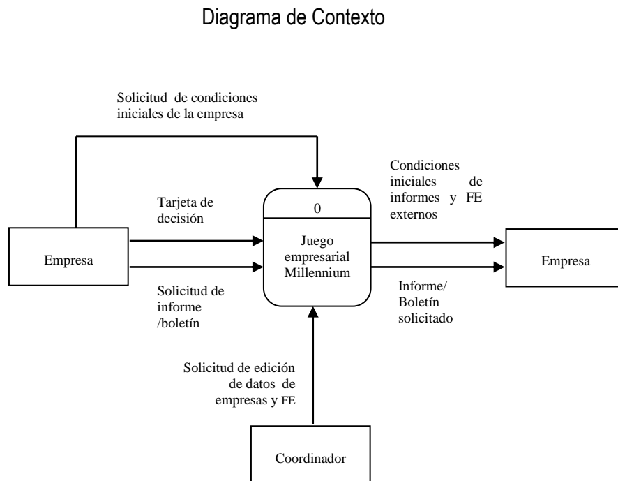
Figura 3. 2 Diagrama de Contexto
