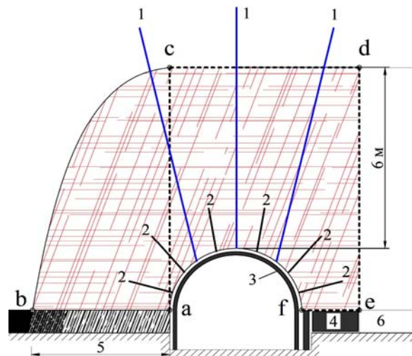
Рисунок 12. Схема нагрузки на крепь выработки за очистным забоем и рекомендуемая схема установки канатных анкеров: 1 – канатный анкер; 2 – штанговый анкер; 3 – рамная крепь; 4 – охранный конструкция; 5 – ширина зона разрушения краевой части пласта (Zabolotnaya, 2015); 6 – выработанное пространство
