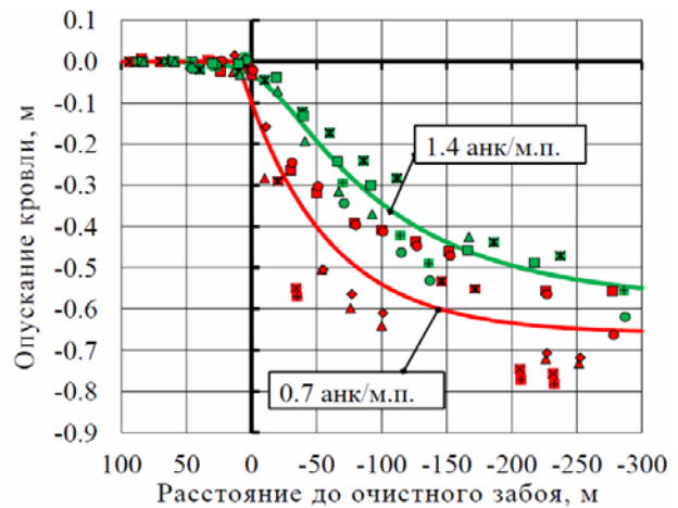
Рисунок 8. Смещения кровли выработки при плотности установки канатных анкеров 0.7 шт/м.п. и 1.4 шт/м.п
