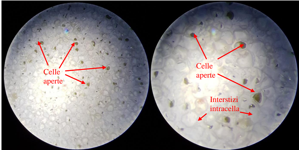
Figura 3: Immagine al microscopio ottico (a sinistra) dello Styrodur usurato, e ingrandimento delle celle danneggiate del polistirene (a destra).
