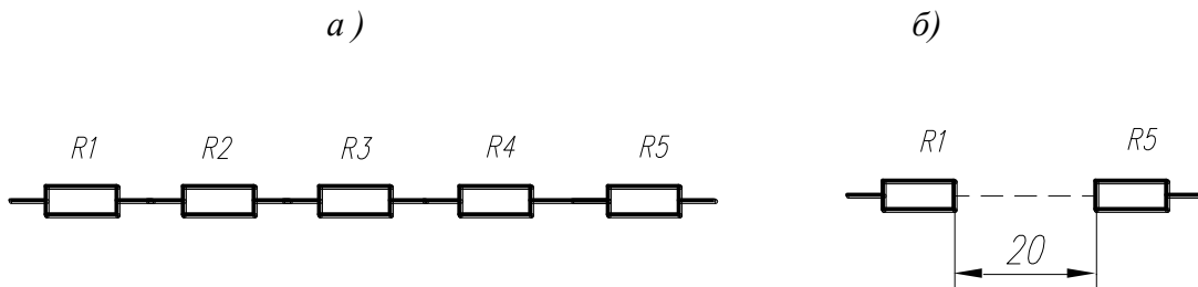
Рис. 2.7. Зображення послідовно сполучених однакових елементів а — дійсне, б — умовне
