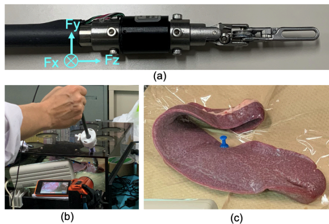
図 1 力覚センサ付き鉗子を用いた摘出臓器に対する押込操作の計測、(a) 力覚センサ付き鉗子の先端付近の外観、(b) 実験環境、(c) 摘出臓器 (脾臓)
