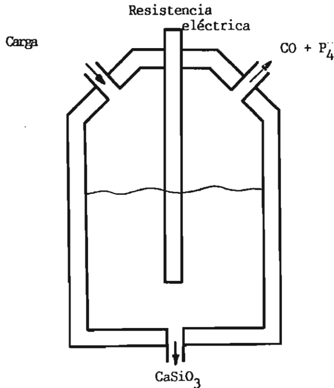
Fig. 2.1 Obtención de fósforo en el horno eléctrico
