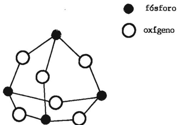
FIG. 4.1 Estructura del óxido fosforoso P_4O_6
