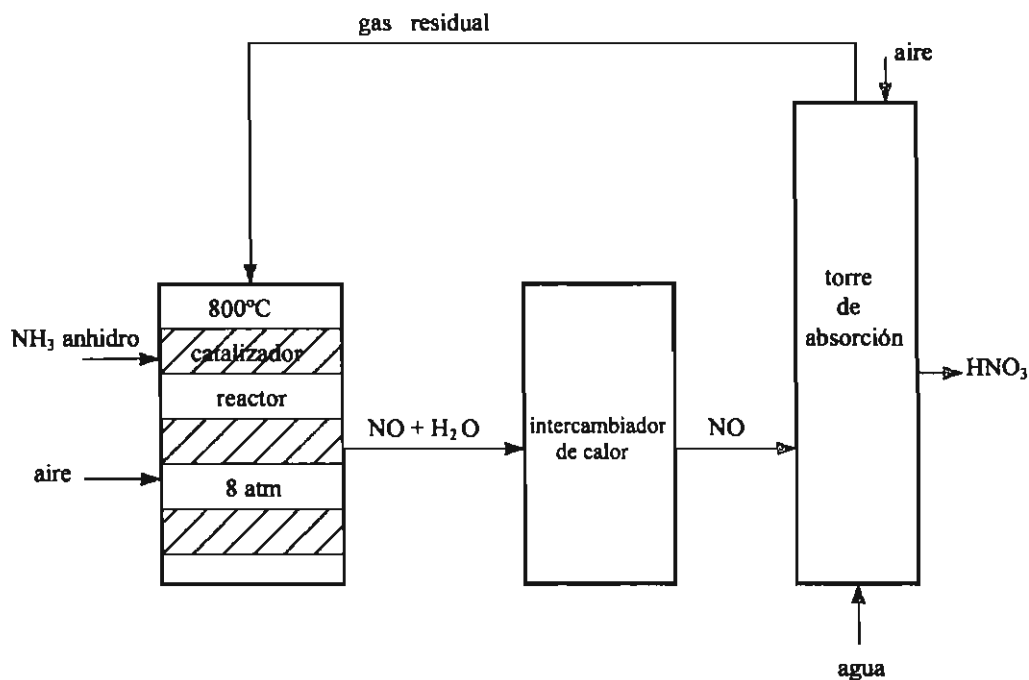
Fig. 6.1. Principio esquemático que ilustra la obtención de ácido nítrico en la industria
