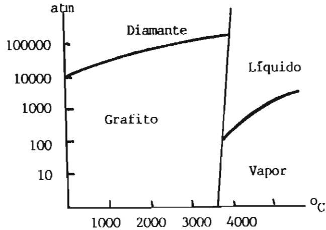
Fig. 1.1 Diagrama de estado del carbono
