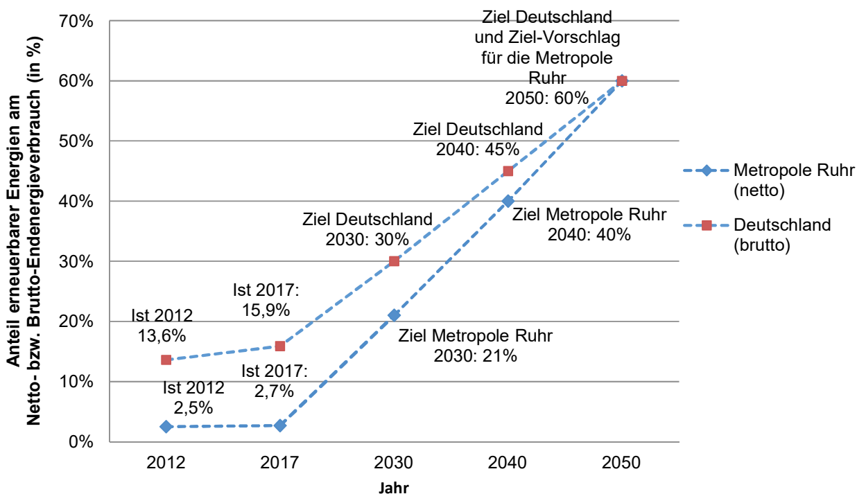
Anteil erneuerbarer Energien am Endenergieverbrauch im Ruhrgebiet (netto) und in Deutschland (brutto) 2012 und 2017 mit Zielen der Bundesregierung und Ziel-Vorschlägen des Wuppertal Instituts für das Ruhrgebiet bis 2050
