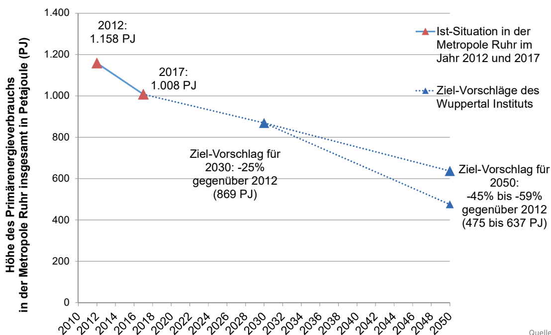
Primärenergieverbrauch in der Metropole Ruhr in den Jahren 2012 und 2017 insgesamt und Ziel-Vorschläge des Wuppertal Instituts für die Jahre 2030 und 2050
