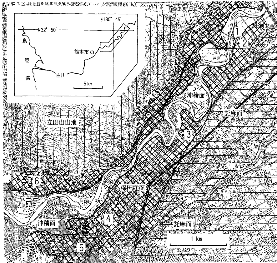
図-1 調査地域位置図および柱状図位置・地形・段丘区分の関係図 地形区分は、託麻面、保田窪面、いわゆる沖積面に3分し、立田山山地も区別して図示した。
