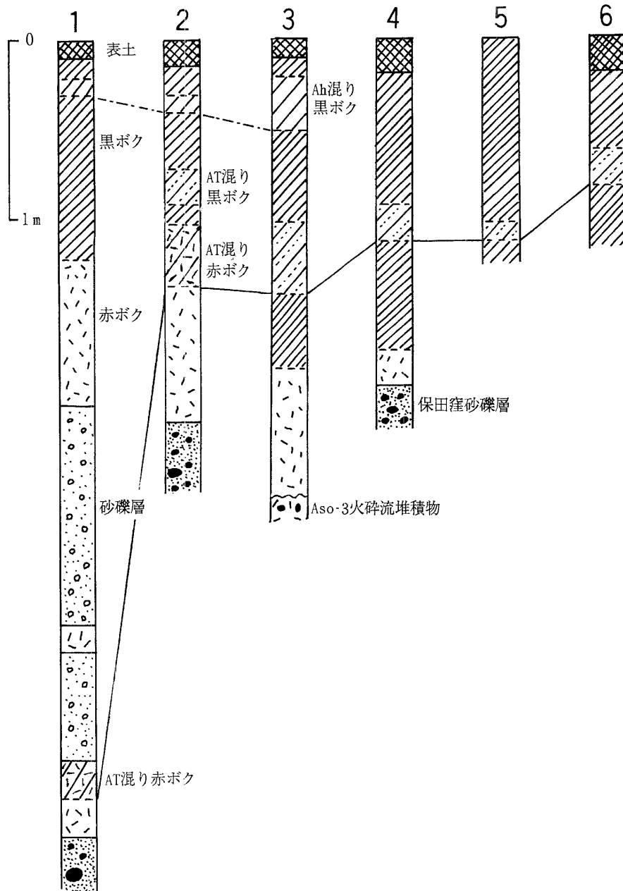
図-2 段丘面構成する堆積物の柱状図 (柱状図の位置は図-1 に示す) 1; 保田窪面より低位の面, 2~6: 保田窪面
