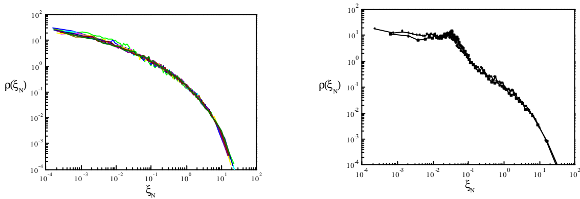
Figure III - 39 : Distribution des forces normales dans différentes couches en échelle logarithmique. A gauche: couches éloignées du socle. A droite, deux premières couches ( N = 1000 - q = 19^\circ - p = 0,15 ).
