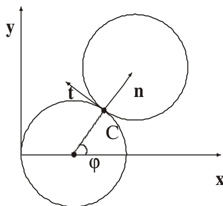
Figure III - 30 : Orientation du contact entre deux grains repérée par un angle \varphi par rapport à la direction d'écoulement ( x'Ox ).
