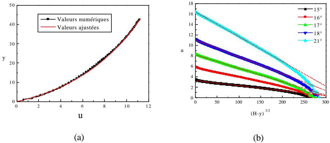
Figure III - 11 : Forme du profil de vitesse.
