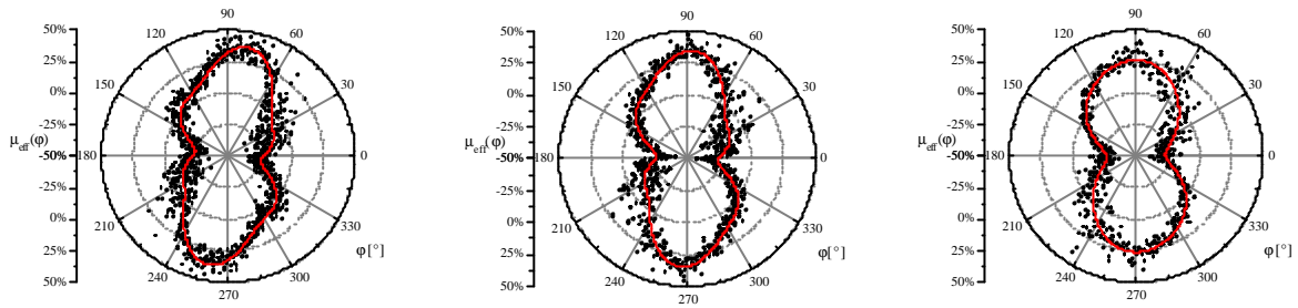
Figure III - 48 : Mobilisation du frottement ( N = 500 - \mathbf{q} = 17^\circ, 22^\circ \text{ et } 26^\circ - p = 0,1 ).
