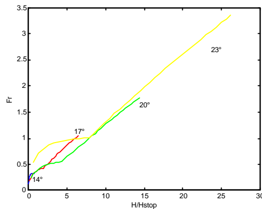
Figure III-18 : Loi d'échelle à partir des paramètres a et b .
