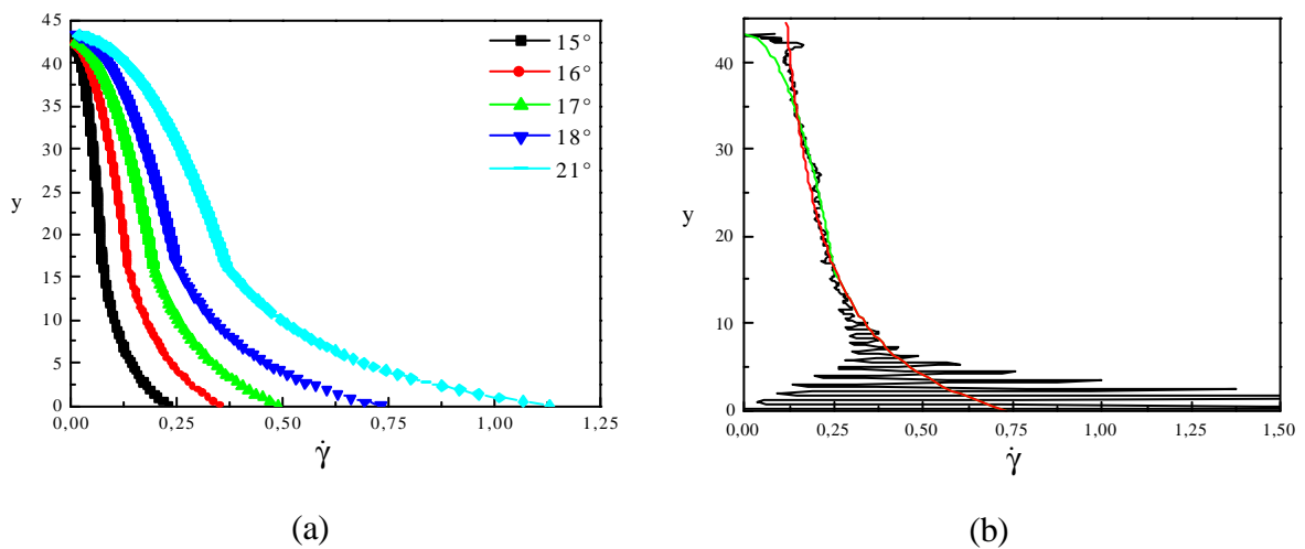
Figure III-12 : a-Profil de taux de cisaillement ajusté selon (III-6 et III-7) pour différentes inclinaisons ( N = 5000 - p = 0.15 ).
