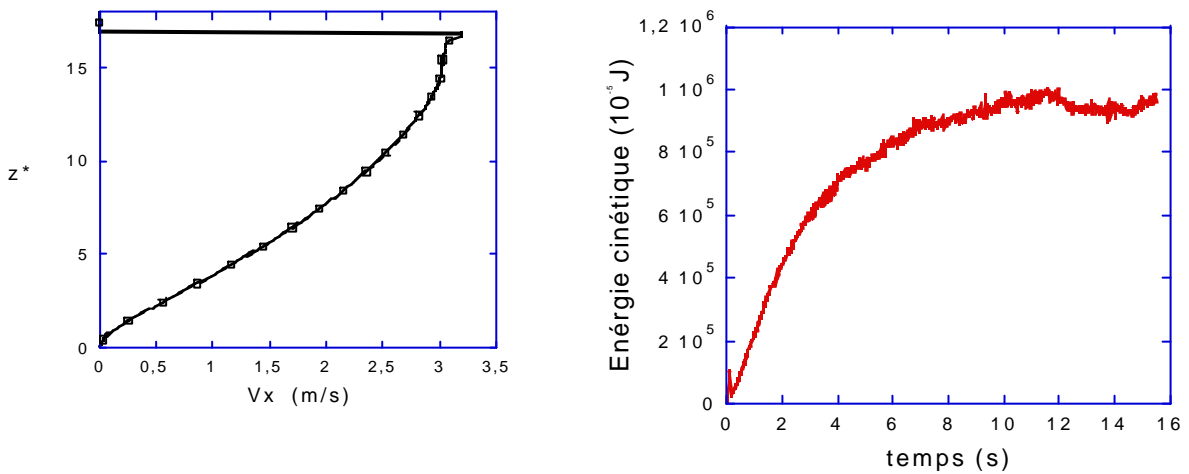
Figure III-60: Profil de vitesse et évolution de l'énergie cinétique pour la simulation d'un écoulement à 33°.
