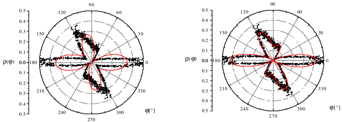
Figure III - 33: Distribution des orientations de contact ( N = 500 - q = 17^\circ - p = 0,1 ). Comparaison avec les développements en série de Fourier d'ordre 2 (à gauche) et 3 (à droite).
