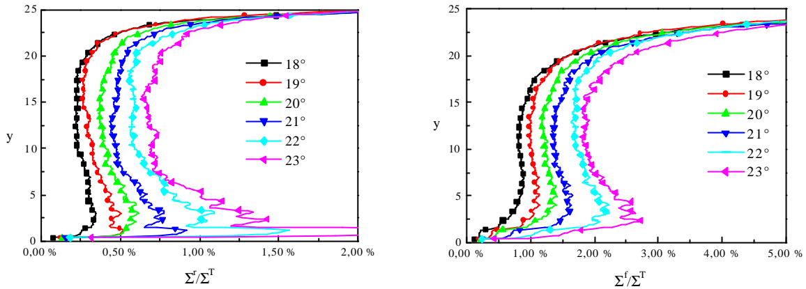
Figure III - 53 : Parties normales des tenseurs de rotation et de Reynolds ( N = 1000 - p = 0,15 ).
