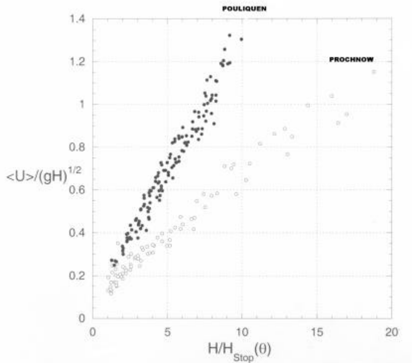
Figure III-16 : Comparaison avec les résultats de Pouliquen.
