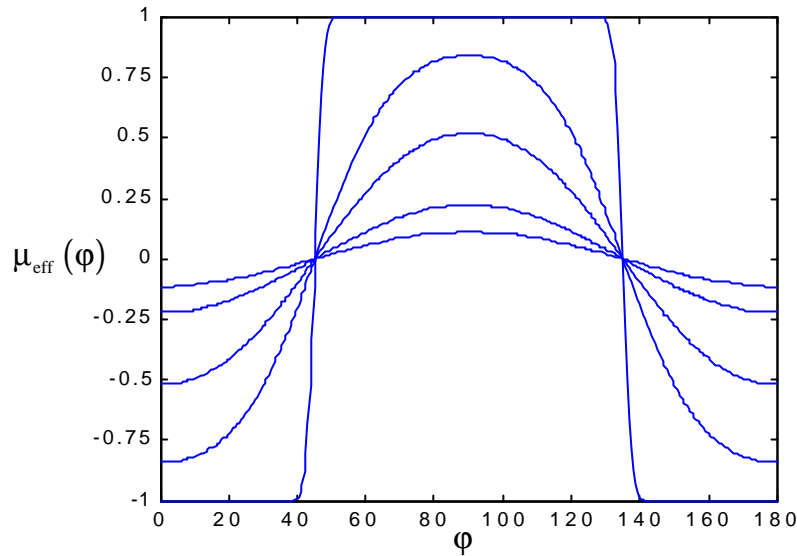
Figure V-16: Prédiction pour m_{eff}(\mathbf{j}) , pour Dw/\langle w \rangle = 10 - 5 - 2 - 1 - 1/10 (distribution gaussienne).
