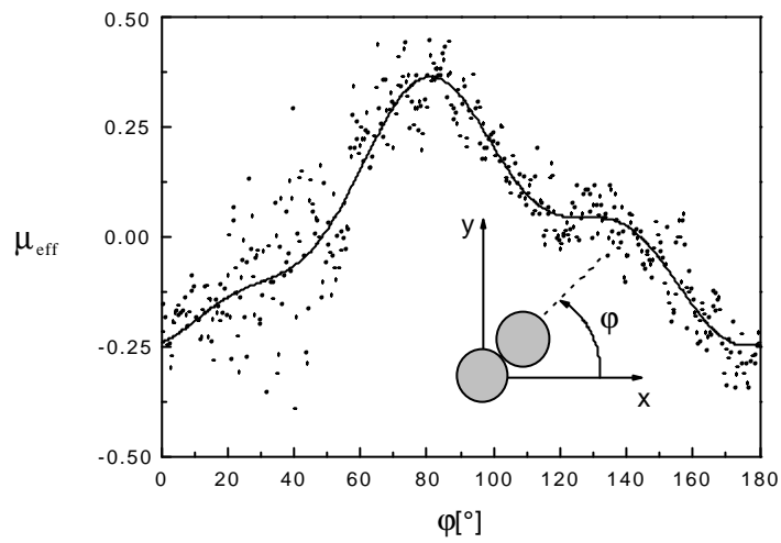
Figure III-49 : Anisotropie de la mobilisation du frottement ( N = 500 - \mathbf{q} = 19^\circ - p = 0 - \mathbf{m} = 0,4 ).
