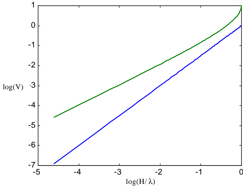
Figure V-9 : Dépendance en H de la vitesse moyenne. On a tracé la dépendance du facteur entre parenthèse de la formule V-67 en fonction de x = H/l . En vert, la dépendance en (H/l)^{3/2} .
