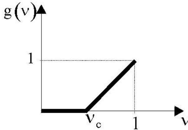
Figure V-5 : Schéma pour la fonction de répartition g(\mathbf{n}) .
