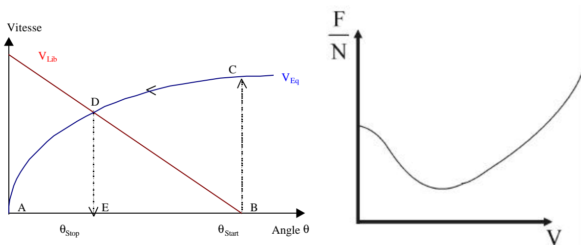
Figure II - 4 : Modèles de Quartier et de Jaeger.
