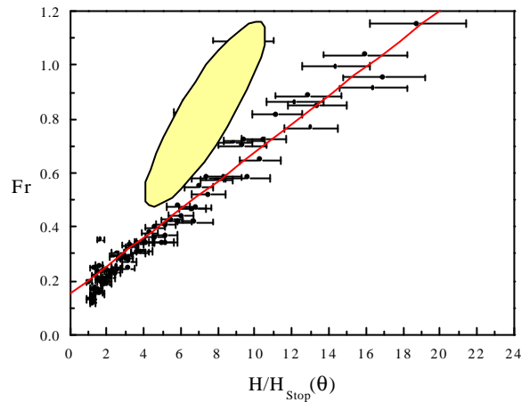
Figure III - 15 : Loi d'échelle faisant intervenir H_{stop}(\mathbf{q}) . La zone jaune correspond aux points H = 40 .
