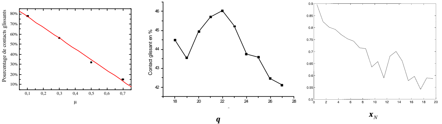
Figure III - 46 : Proportion de contacts glissants en fonction a. du coefficient de frottement ( N = 500 - p = 0 ) b. de l'inclinaison ( N = 1000 - m = 0,4 - p = 0,15 ), c. de l'intensité de la force normale ( N = 500 - m = 0,4 - p = 0 ).
