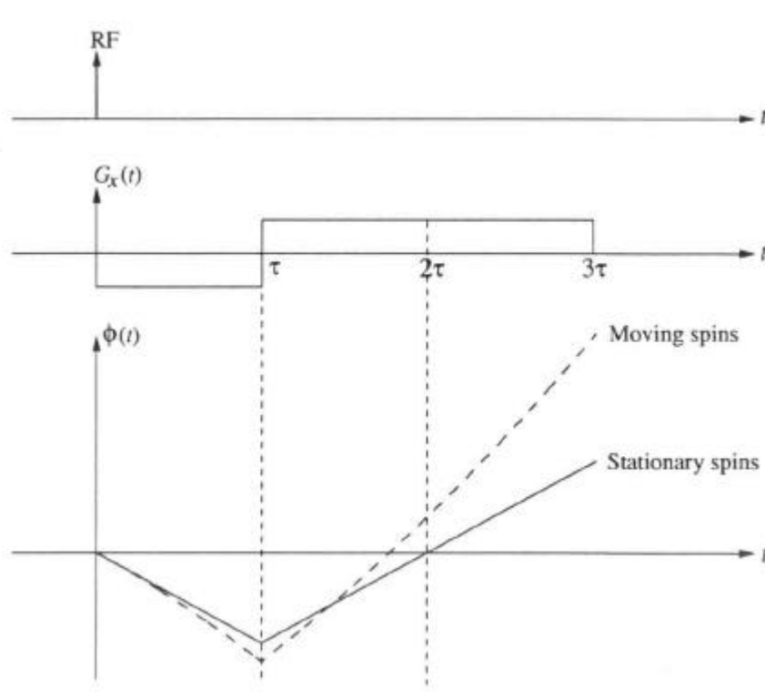
Figure 2-17 : Séquence bipolaire.
