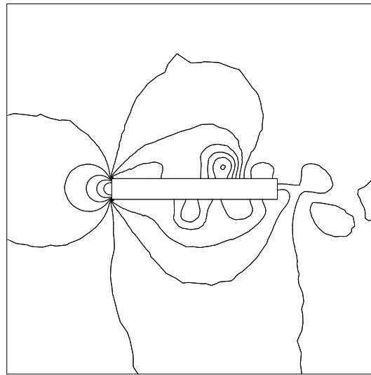
FIG. 34 – Lignes d'isopression autour du tablier, u=12m/s , t=0.6s
