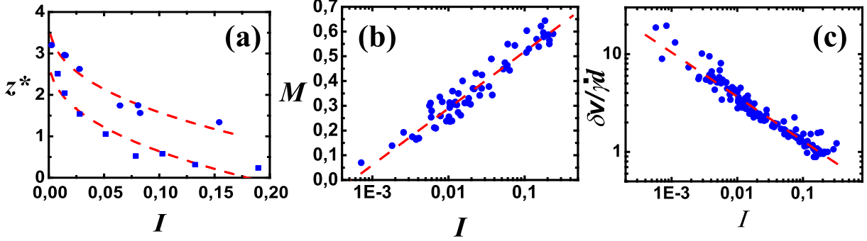
FIG. 15 – Cisaillement plan - Aspects microstructurels (a) Nombre de coordination pour \mu = 0 (disques bleus, e_N = 0.1 - carrés bleus : e_N = 0.9 ) ; (b) Mobilisation du frottement ; (c) Fluctuations relatives de la vitesse de translation.
