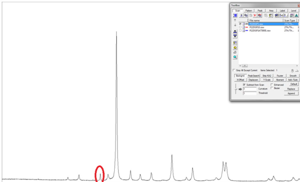
Ilustración 99 P22 grava fina dolomitas microondas 5 min
