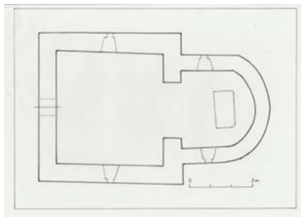
63. kép. A Szent Mihály kápolna I. és II. periódusának alaprajza
