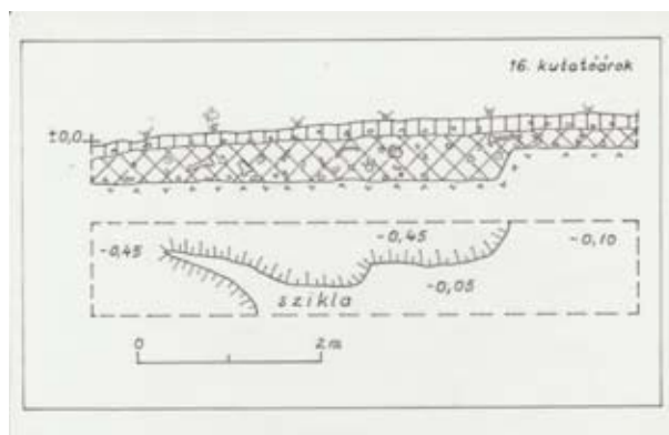
47. kép. A 16. kutatóárok alaprajza és metszete
