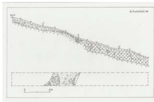
43. kép. A 6. kutatóárok alaprajza és metszete
