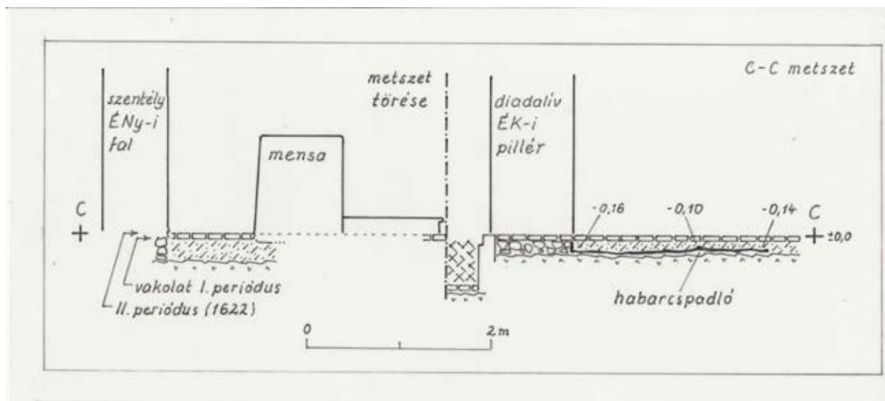
30. kép. C–C metszet
