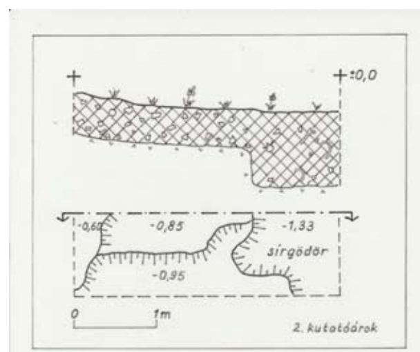
29. kép. A 2. kutatóárok alaprajza és metszete
