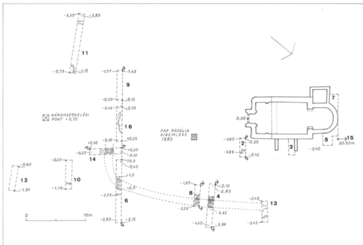
33. kép. A Szentmihály-dombon végzett ásatás összesített alaprajza
