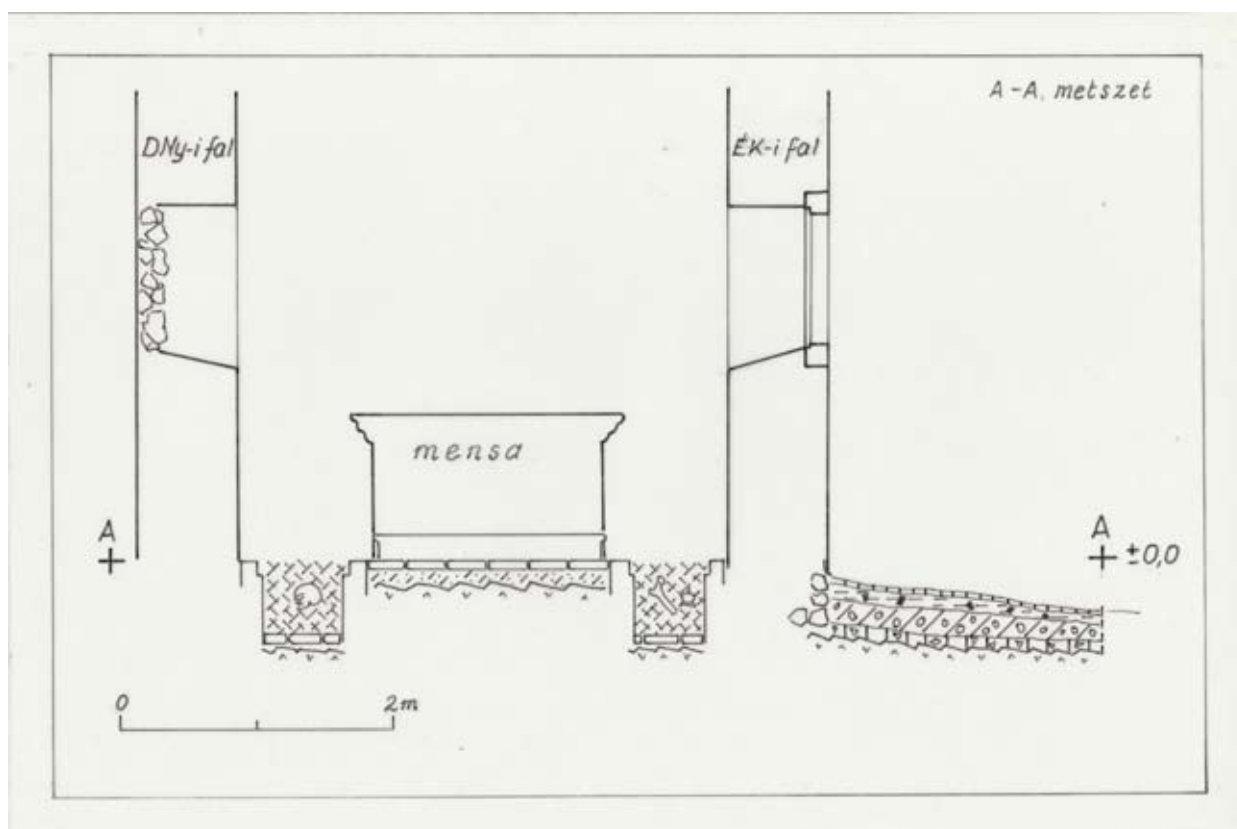
27. kép. A–A metszet
