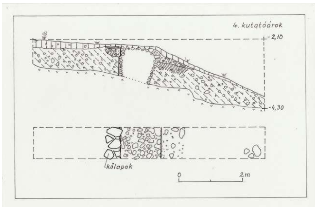
37. kép. A 4. kutatóárok alaprajza és metszete
