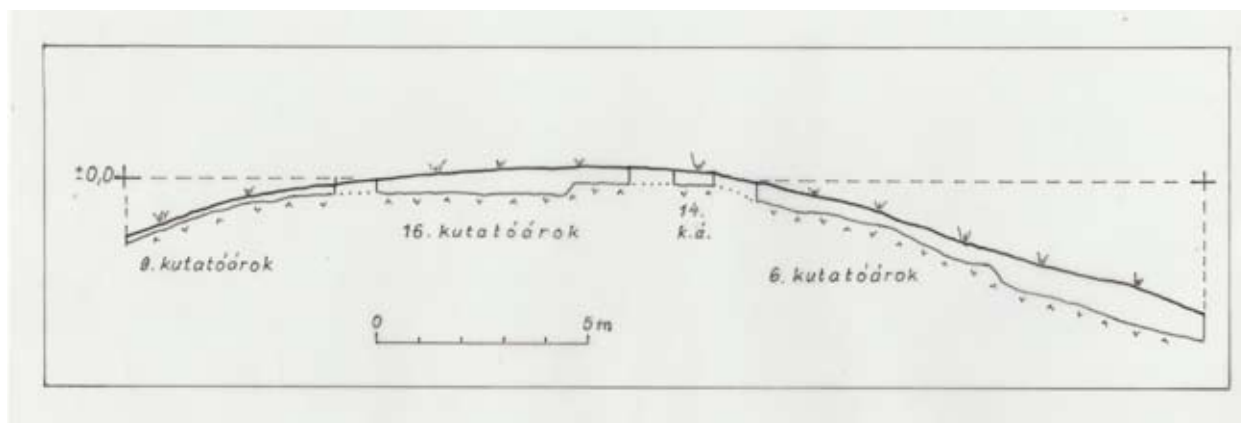
45. kép. A dombtető metszetrajza
