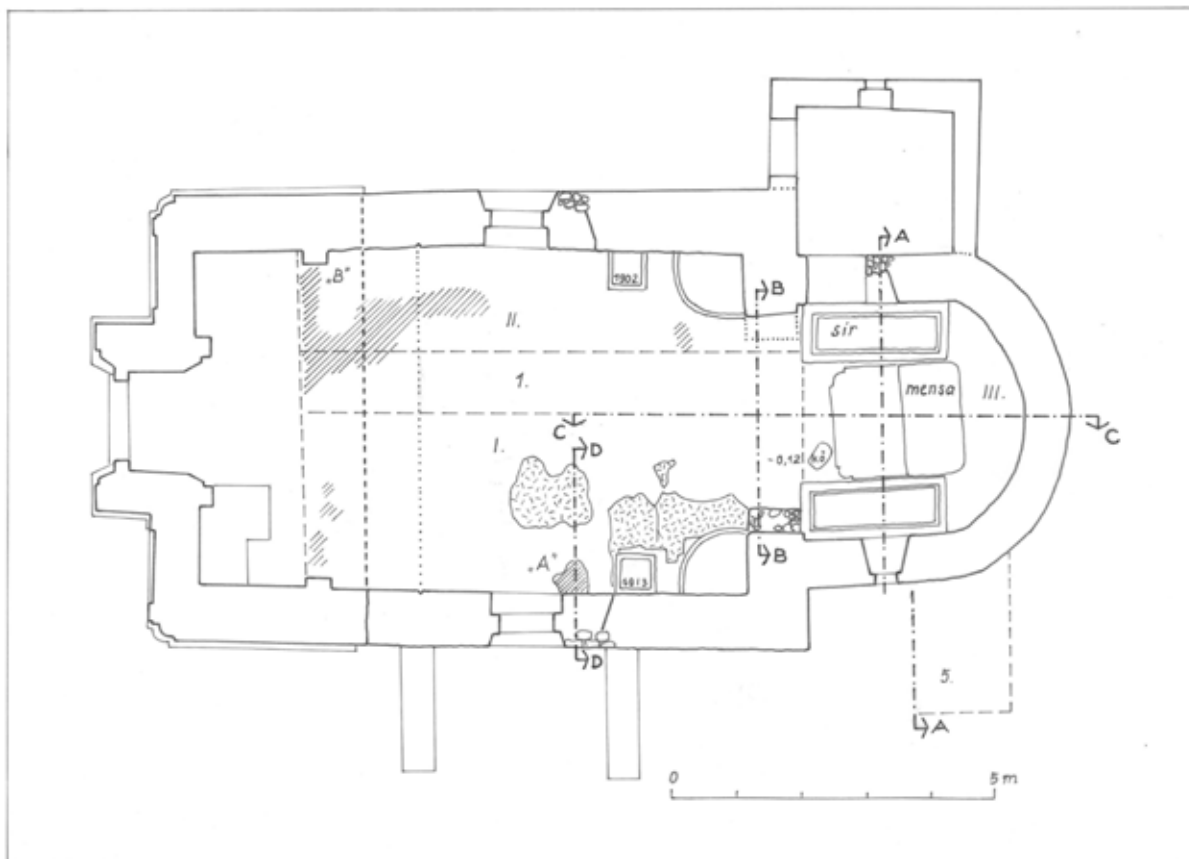
19. kép. A Szent Mihály kápolna ásatási alaprajza a metszetek helyével
