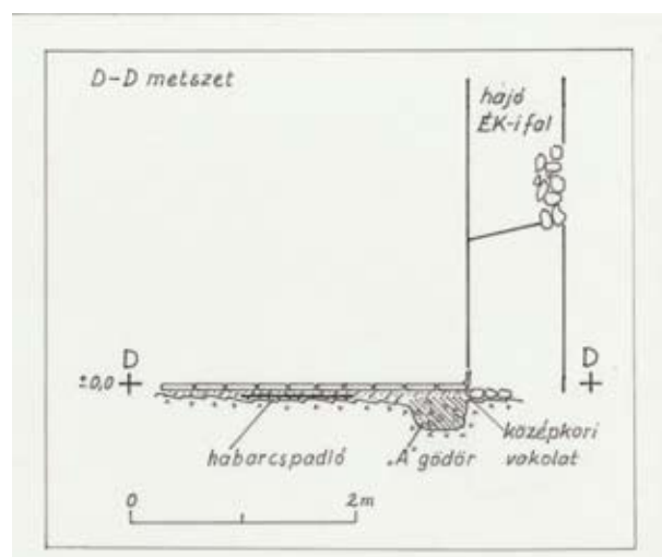
32. kép. D–D metszet
