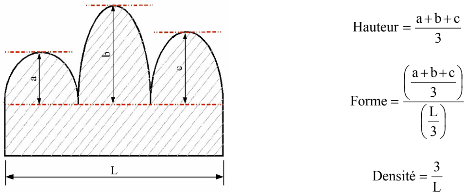
Figure II.4 : Définition des descriptions de taille, forme et densité
