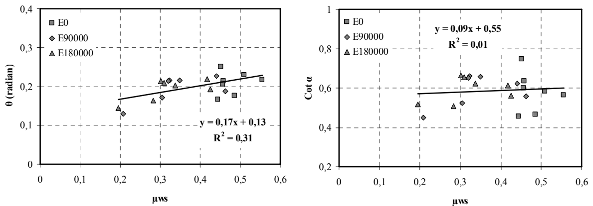
Figure V.20 : Évolutions des paramètres \theta et \text{Cot } \alpha en fonction du frottement dans le cas de l'ensemble des granulates (Profil seuillé, Échelle de rugosité)
