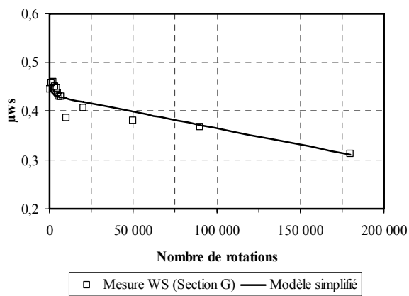
Figure VIII.60 : Courbes d'évolution comparées : mesures et modèle simplifié « LCPC » (site de Fontenay, PSV = 50)
