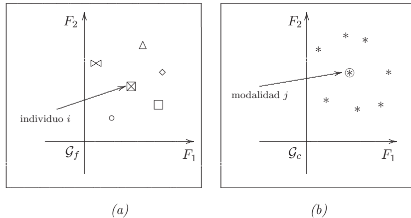
Figura 11.9 Proyección de individuos y modalidades
