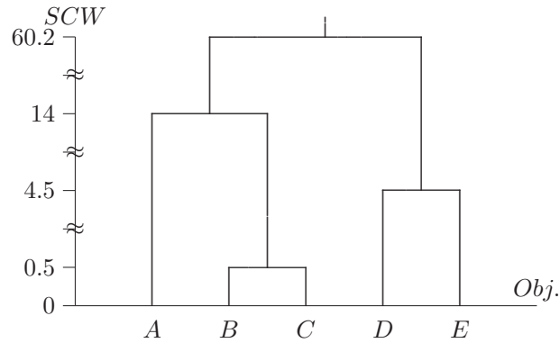
Figura 7.5 Dendrograma: método de la SC de Ward.
