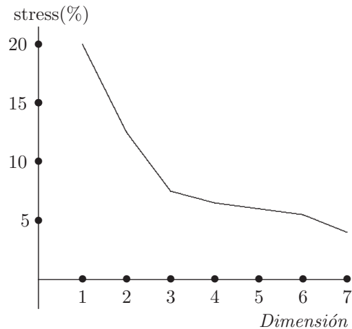
Figura 10.5 Selección de la dimensionalidad.
