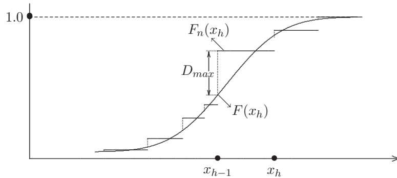
Figura 2.2 Contraste de Kolmogorov-Smirnov.
