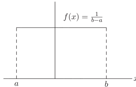
Figura B.2 Distribución uniforme.
