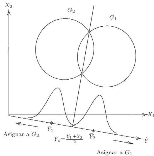
Figura 8.1 Discriminación lineal.
