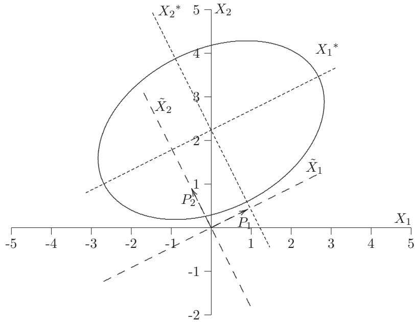
Figura A.5 Translación y rotación.
