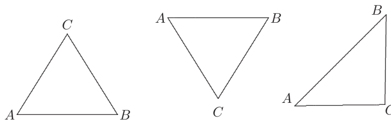
Figura 10.1 Mapa de la similitud entre tres objetos.
