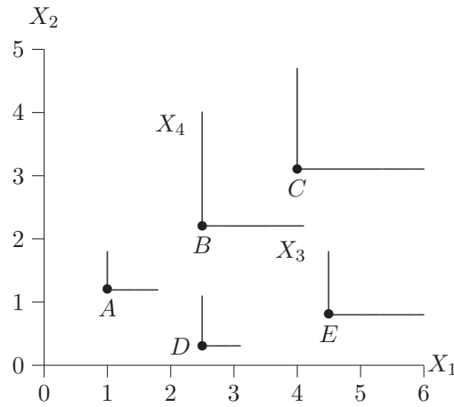
Figura 1.2 Gráfico para cuatro dimensiones.
