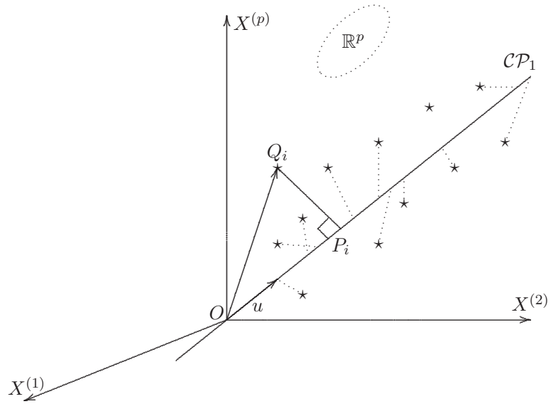
Figura 5.5 Proyección sobre una línea recta.
