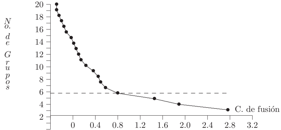
Figura 7.11 Número de grupos vs coeficiente de fusión.
