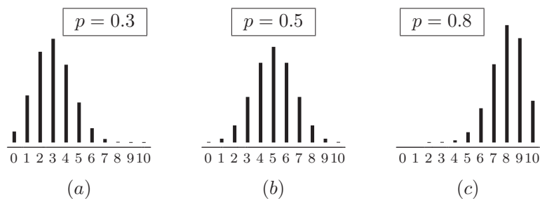
Figura B.5 Distribución binomial.
