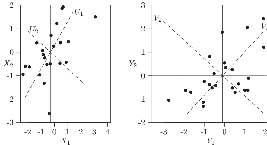
Figura 9.2a Variables canónicas en \mathbf{X} . Figura 9.2b Variables canónicas en \mathbf{Y} .
