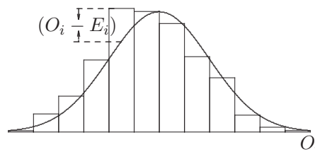
Figura 2.1 Contraste Ji-cuadrado para normalidad.
