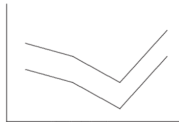
Figura 3.7b Hipótesis H_{02} falsa.
