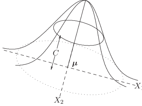
Figura 2.5 Densidad constante en una normal bivariada.
