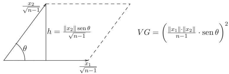
Figura 1.8 Varianza generalizada.
