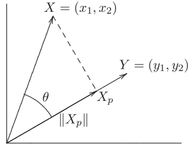
Figura A.1 Proyección ortogonal.
