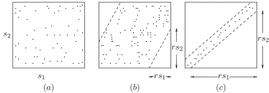
Figura 1.9 Desviación típica generalizada.
