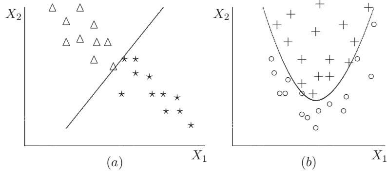
Figura 8.3 Discriminación: (a) lineal, (b) cuadrática.
