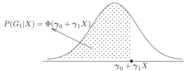
Figura 8.6 Discriminación probit.
