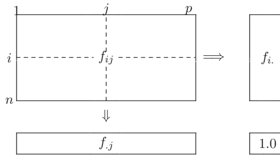
Figura 11.1 Tabla de frecuencias y sus marginales.
