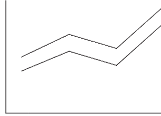
Figura 3.9b Hipótesis H_{03} falsa.
