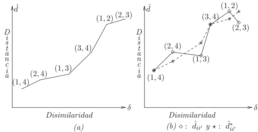
Figura 10.4 Diagramas de Shepard.
