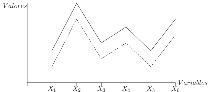
Figura 7.1 Perfiles con coeficiente de correlación r = 1.0 .
