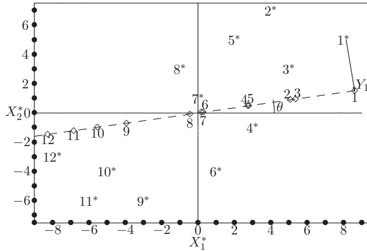
Figura 5.1 Datos corregidos (*) y proyectados sobre Y_1 ( \diamond ).
