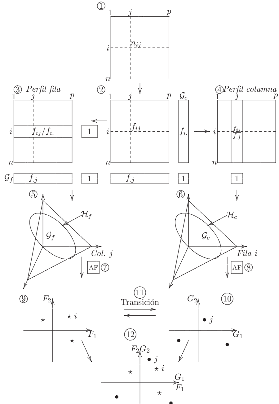
Figura 11.6 Esquema del análisis de correspondencias 2 .
