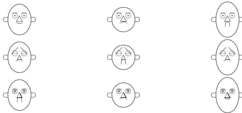
Figura 7.8 Rostros de Chernoff.
