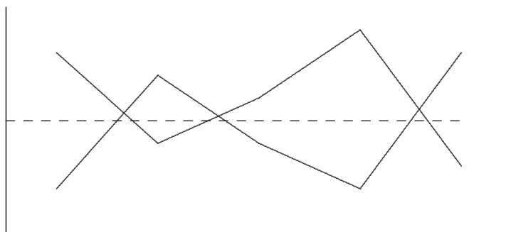
Figura 3.8 Hipótesis H_{02} : “igual efecto sin paralelismo”.
