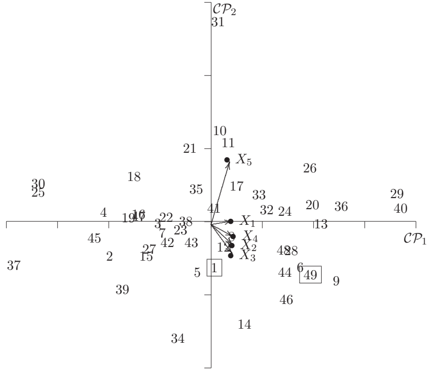
Figura 5.12 Biplot para el ejemplo 5.1.
