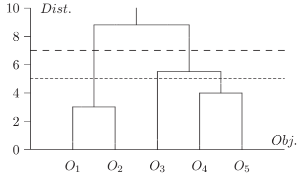
Figura 7.4 Dendrograma: método del promedio.
