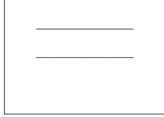
Figura 3.9a Hipótesis H_{03} verdadera.
