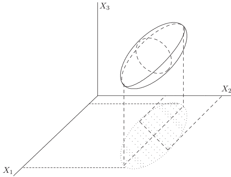
Figura 3.3 Región de confianza.
