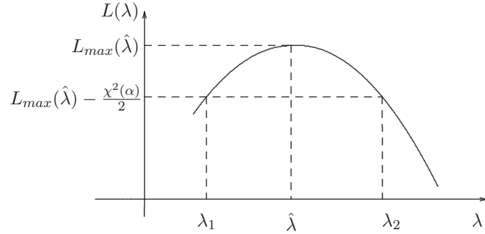
Figura 2.3 Estimación gráfica de \lambda .
