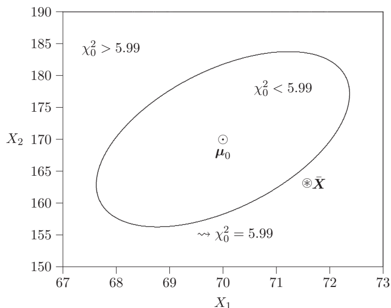
Figura 3.1 Región de no rechazo bivariable.
