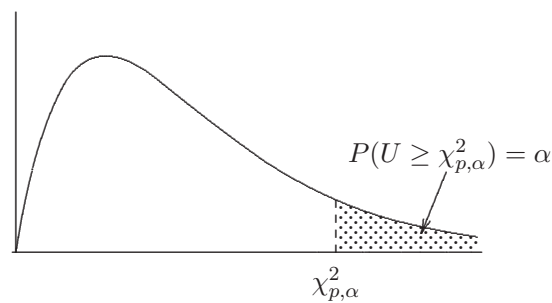
Figura B.4 Distribución ji-cuadrado.
