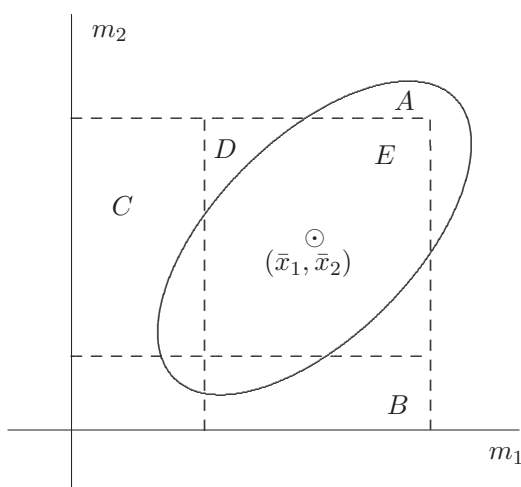
Figura 3.4 Región de confianza bivariada.
