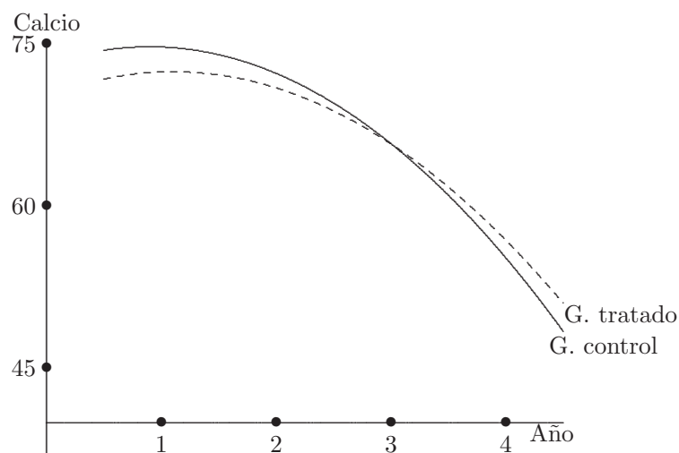
Figura 3.11 Curvas de crecimiento, grupo control y tratamiento.
