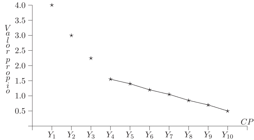
Figura 5.8 Selección del número de componentes principales.
