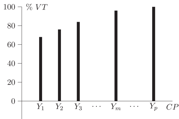
Figura 5.7 Variación retenida hasta cada componente principal.
