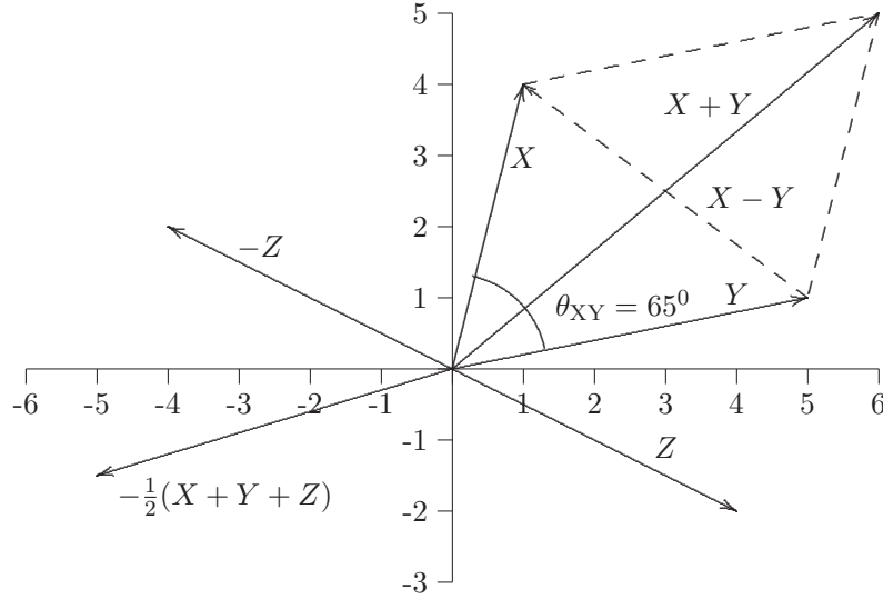
Figura A.2 Operaciones entre vectores.
