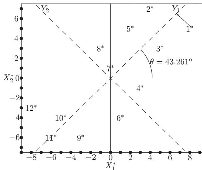
Figura 5.3 Datos corregidos (*) y nuevos ejes.
