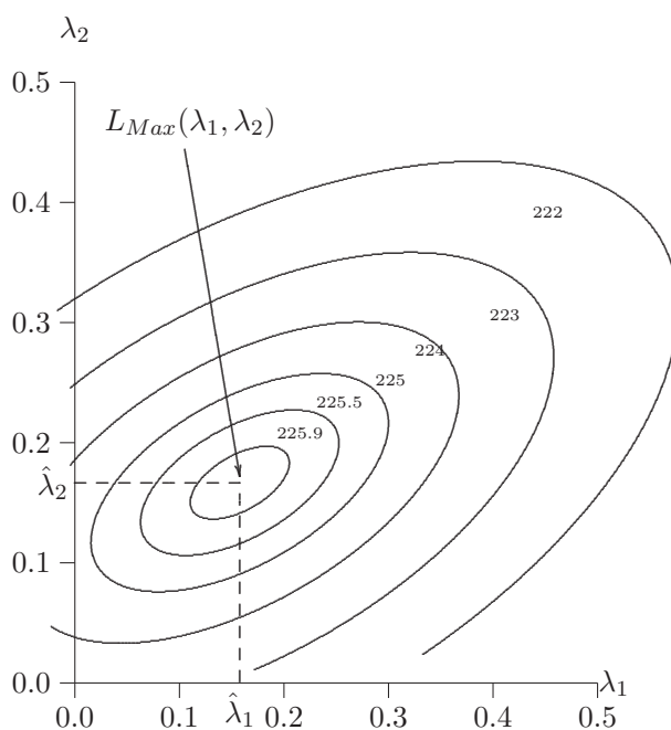
Figura 2.4 Curvas de nivel para L(\lambda_1, \lambda_2) con los datos de radiación.
