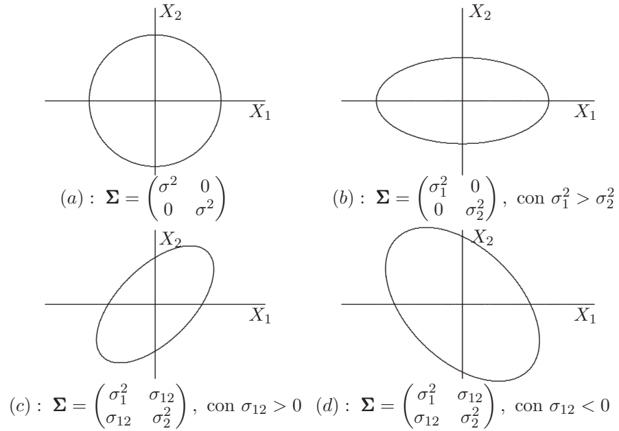
Figura 4.1 Elipses asociadas con la matriz de covarianzas.
