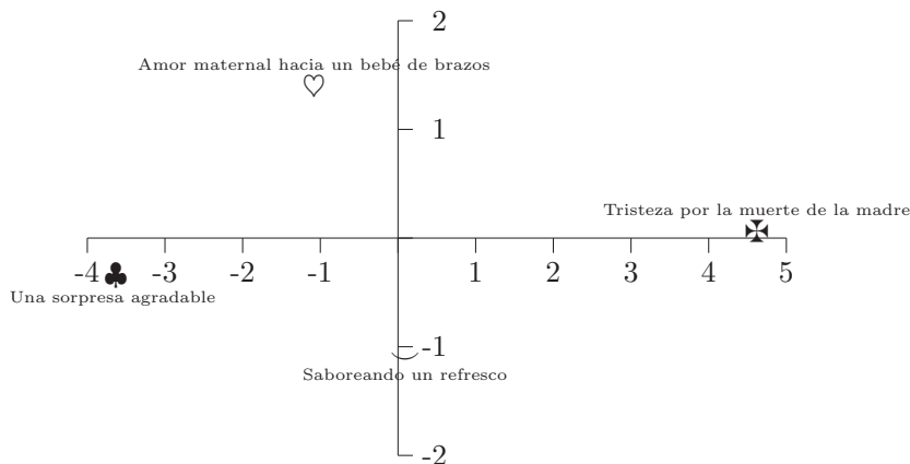
Figura 10.3 Posicionamiento de las cuatro expresiones faciales.
