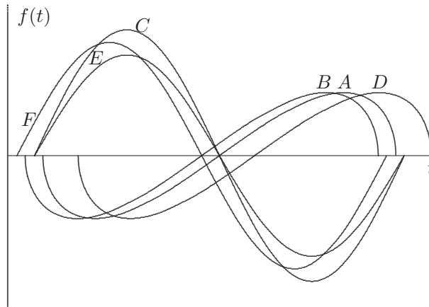
Figura 7.9 Curvas de Andrews para clasificar seis objetos.
