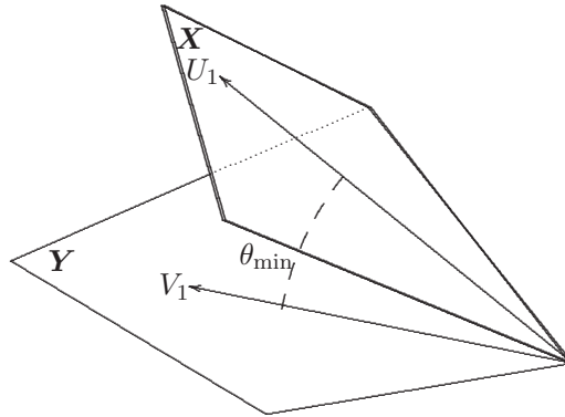
Figura 9.3 Esquema geométrico del análisis de correlación canónica.
