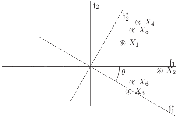
Figura 6.2 Rotación de factores.
