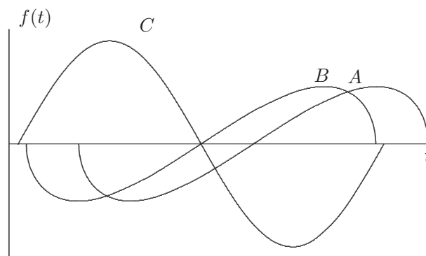
Figura 1.7 Curvas de Andrews.
