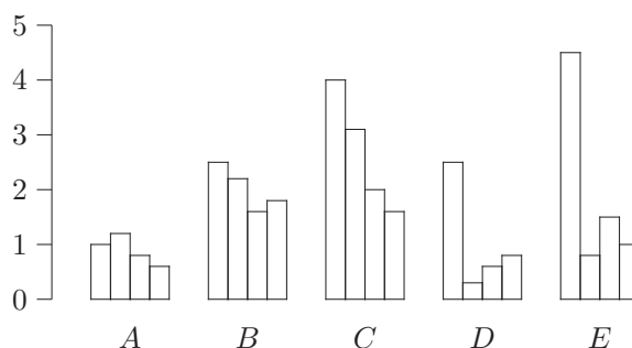
Figura 1.3 Perfiles de la matriz de datos X .
