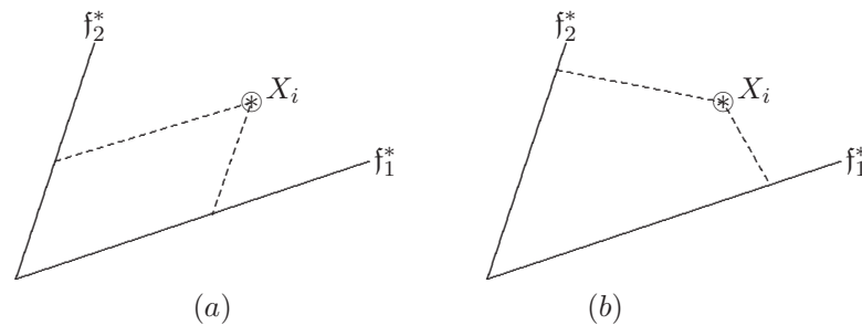
Figura 6.3 Rotación oblicua de factores.
