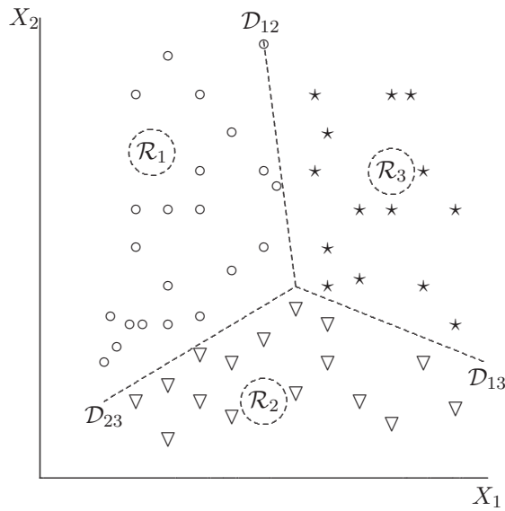
Figura 8.4 Regiones de discriminación para tres grupos.
