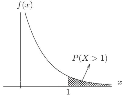
Figura B.1 Función de densidad.
