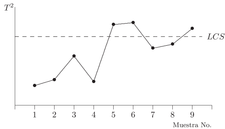
Figura 3.5 Carta de control T^2 .
