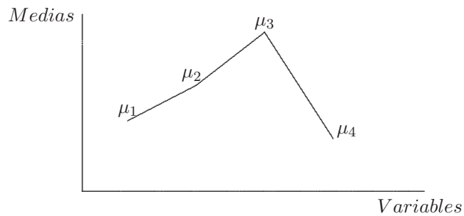
Figura 3.6 Perfil de medias, p = 4 .
