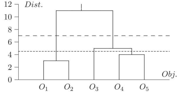
Figura 7.3 Dendrograma: método del vecino más lejano.
