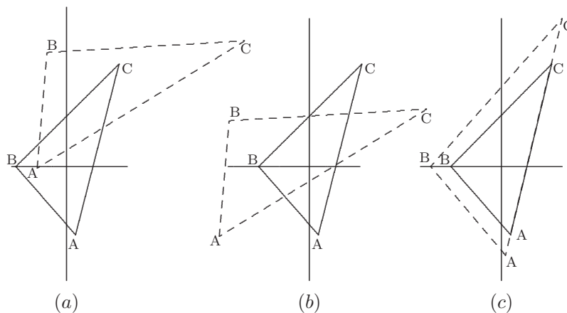
Figura 10.6 Método de acoplamiento (Procrusto).
