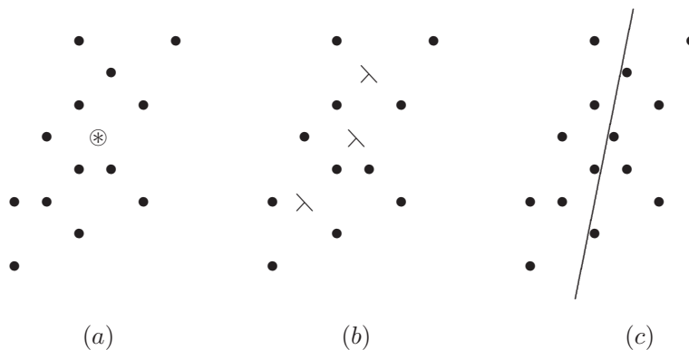
Figura 7.6 Núcleos: (a) Centroides, (b) Individuos y (c) Recta.
