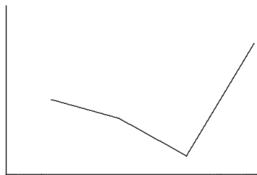
Figura 3.7a Hipótesis H_{02} verdadera.
