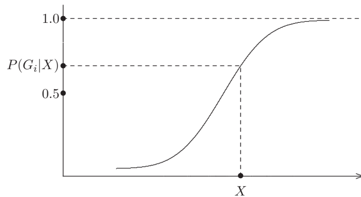
Figura 8.5 Función logística.
