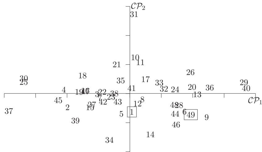
Figura 5.10 Primer plano factorial.
