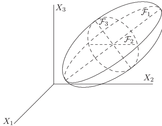
Figura 5.6 Componentes principales bajo normalidad.
