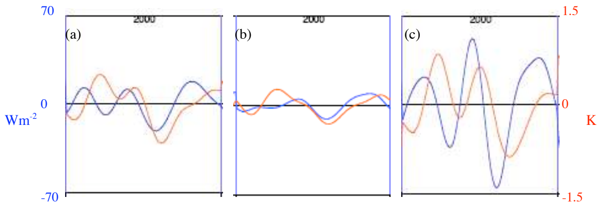
Figure 2.14 Signaux reconstruits sur janvier, février et mars 2000, d'OLR (bleu, Wm^{-2} ) et de TSO (reprojeté sur l'OLR, rouge, °C) pour les deux premières composantes principales réelles (a), la première composante principale complexe (b) comparés aux signaux d'entrées (c) pour la région 72.5^{\circ}E-10^{\circ}S .
