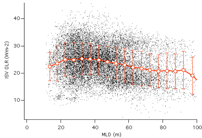
Figure 3.6 Amplitudes moyennes mensuelles de la variabilité intrasaisonnière de l'OLR en fonction de la profondeur de la couche de mélange océanique pour chaque région de 2,5^\circ \times 2,5^\circ pour laquelle la moyenne de l'OLR est inférieure à 250 \text{ Wm}^{-2} (régions « convectives »).
