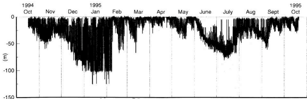
Figure 3.9 Estimation de la profondeur de la couche de mélange océanique en mètres d'après les mesures effectuées par le mouillage du Woods Hole Oceanographic Institution (WHOI) à 61.5° Est, 15,5° Nord. Figure issue de McCreary et al (2001).
