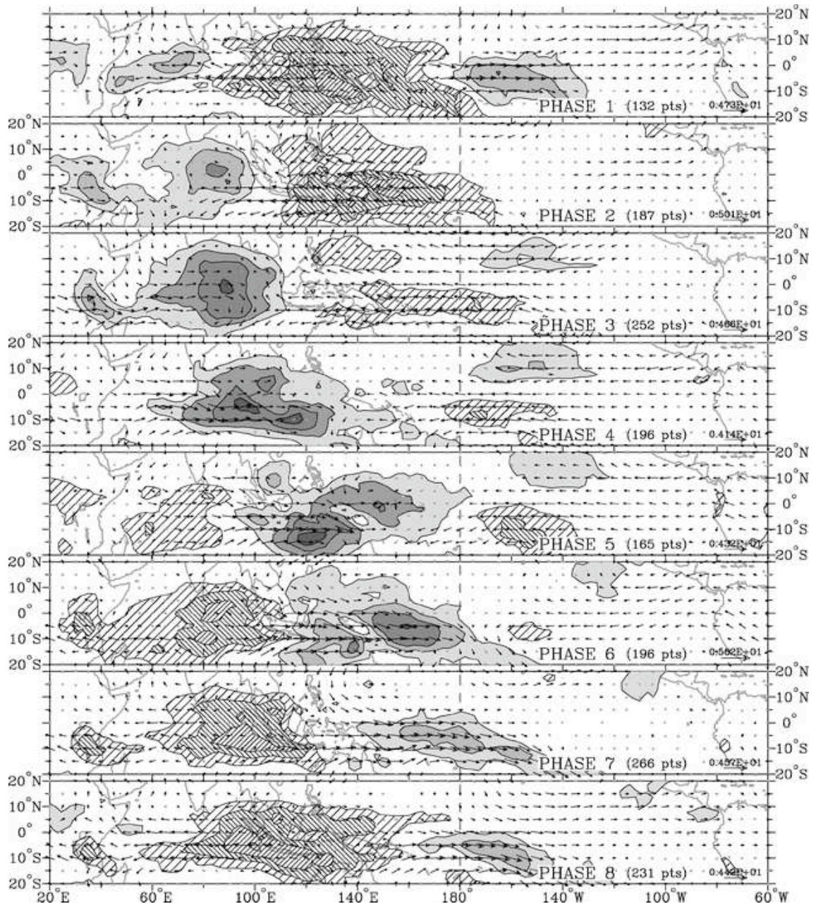
Figure 1.4 Composite d'OMJ pendant décembre-février 1979-2001 pour l'OLR (NOAA) et le vent à 850 hPa (NCEP). Le composite est basé sur un indice symétrique par rapport à l'équateur ( -15^{\circ} à 15^{\circ} Nord), les grisés correspondent à des anomalies de -7.5 , -15 , -22.5 et -30 \text{ Wm}^{-2} (soit un renforcement de la convection) et les parties hachurées à des anomalies de 7.5 et 22.5 \text{ Wm}^{-2} . D'après Wheeler et Hendon (2004).
