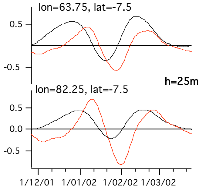
Figure 4.27 Evolutions régionales reconstruites des perturbations de TSO en rouge (événement de l'hiver 2002) et perturbation potentielle de TSO pour une couche mélangée de profondeur h=25m calculée à partir de la perturbation de flux à la surface liée aux perturbations convectives associées à l'événement de TSO de l'hiver 2002 en noir.
