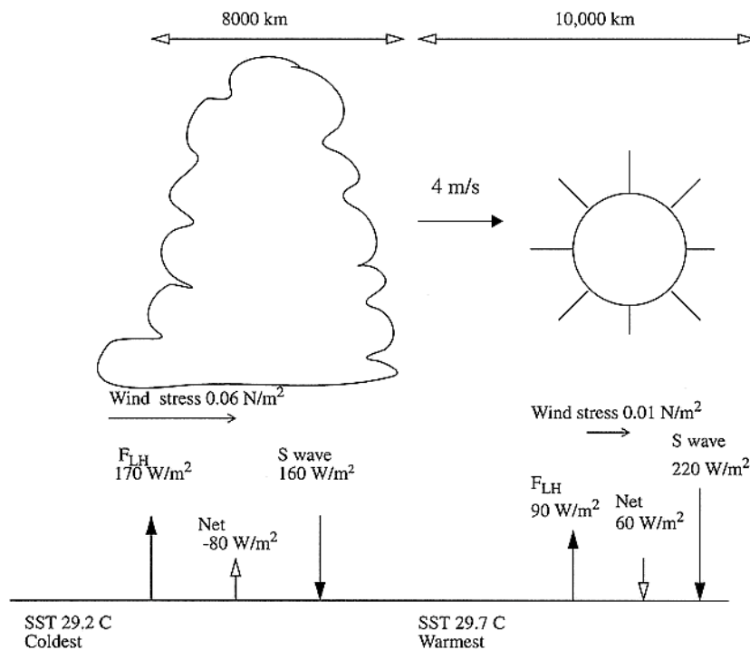
Figure 1.15 Diagramme schématisé zonal des amplitudes et relations de phases observées relativement à la perturbation convective des flux de surface et de la température de surface de l'océan pour une variation intrasaisonnière se propageant vers l'Est à 4\text{ms}^{-1} dans le Pacifique Ouest (OMJ). D'après Shinoda et al (1998).
