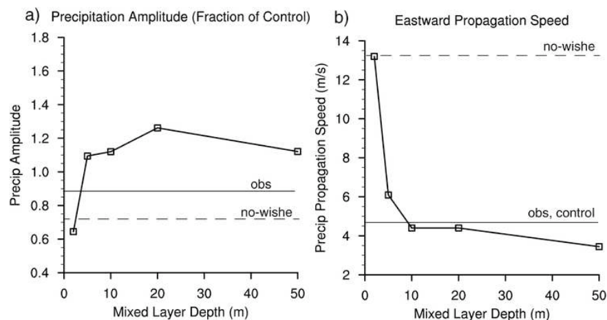
Figure 3.1 (a) Ecart types pour et (b) vitesse de propagation vers l'Est des variations intrasaisonnières de la précipitation dans le MCG du National Center for Atmospheric Research (NCAR) entre -10° et 10° Nord et 105° et 165° Est en fonction de la profondeur de la couche de mélange. L'amplitude des variations de précipitation est une fraction de celui pour le modèle forcé par les TSO climatologiques. D'après Maloney et Sobel (2004).
