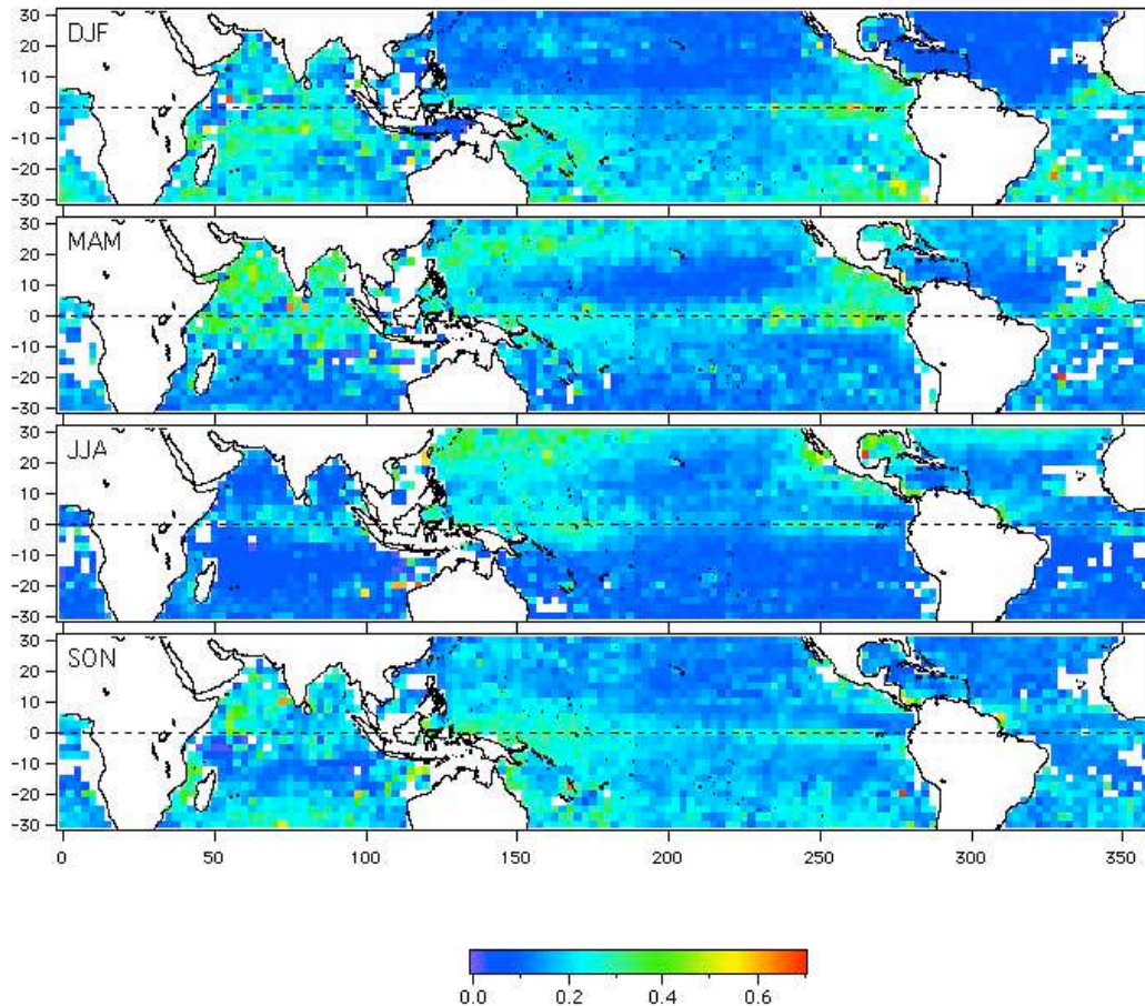
Figure 5.17 Moyennes conditionnelles trimestrielles des cycles diurnes des bouées SVP « Krig » corrigées sur 1979-2002 en K, c'est-à-dire uniquement sur les jours pendant lesquels une bouée est présente sur la région.
