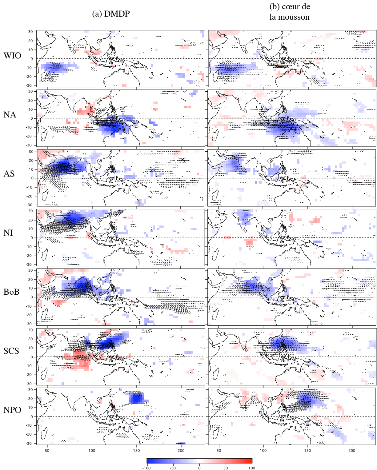
Figure 3.13 Composites des anomalies entre les dates de minimum d'OLR (filtré) d'un fort intrasaisonnier et les dates de maximum précédentes, pour l'OLR brut (moyenné sur 5 jours, en Wm^2 , couleurs) et le vent à 850 hPa brut (moyenné sur 5 jours, 1^\circ=1ms^{-1} ) pour (a) les forts évènements intrasaisonniers associés à la DMDP et (b) pour les forts évènements intrasaisonniers du reste de la saison de mousson (voir figure 10) pour chaque région. Seules les anomalies significatives à 95% sont représentées.
