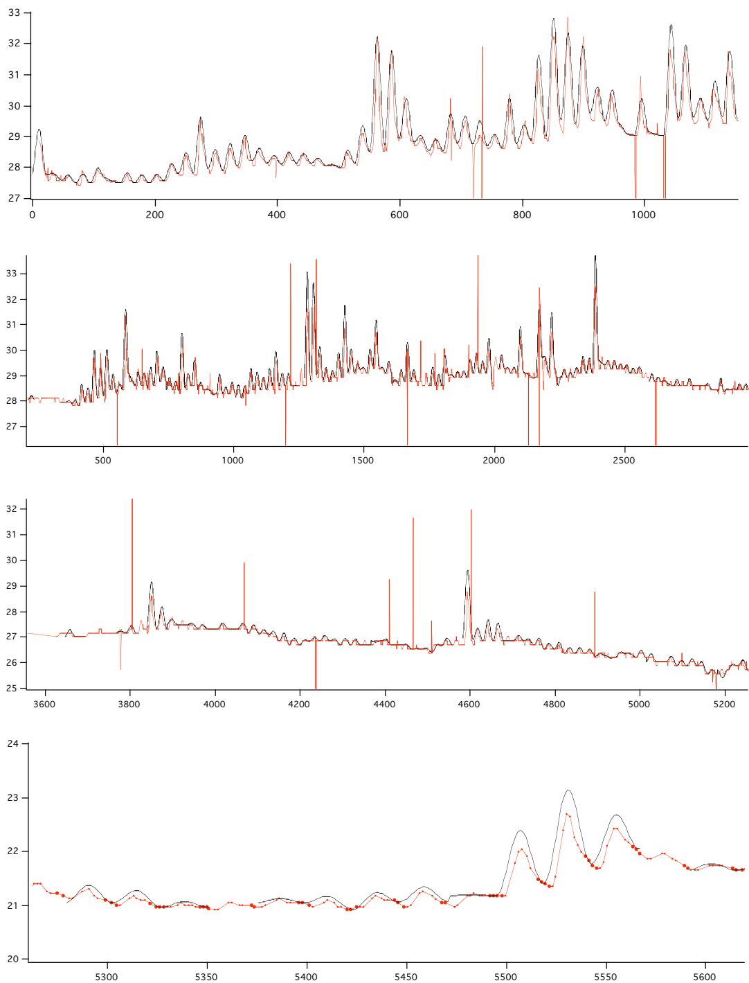
Figure 5.13 Résultats d'interpolations (noir) à partir des données brutes (rouge) pour les bouées 34156 (a) et 2931 (b et c) et 29717 (d). Pour la dernière bouée, les points correspondent aux mesures, les mesures nocturnes sont repérées en gras.
