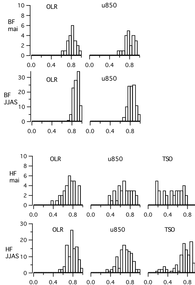
Figure 4.20 Distances à l'événement moyen de mai et de juin-septembre observé des événements des ensembles BF et HF.
