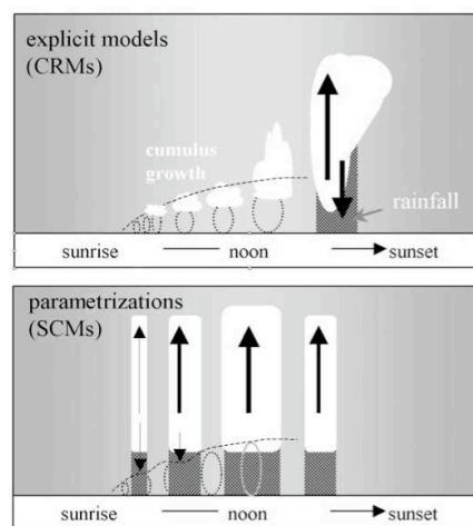
Figure 6.7 Schéma d'évolution diurne de la convection dans un Cloud Resolving Model (en haut) et une colonne de Modèle de Circulation Générale (Single Column Model) , d'après Guichard et al (2004).
