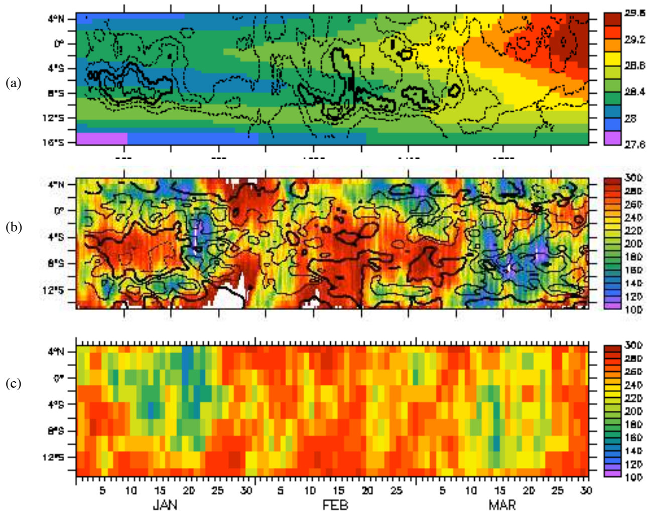
Figure 6.6 Hoevmöller (moyenne entre 60° et 80° Est) de (a) la température BF (couleurs, °C) et la différence entre TDI et TBF (à partir de -0.3^{\circ}\text{C} tout les 0.1^{\circ}\text{C} , la ligne 0^{\circ}\text{C} est en gras, les valeurs négatives en pointillés), (b) l'OLR de la simulation TBF (couleurs, en \text{Wm}^{-2} ) et différence entre les OLR des simulations TDI et TBF (de -5 à 10 \text{ Wm}^{-2} , tous les 5 \text{ Wm}^{-2} ), (c) OLR NOAA (couleurs, en \text{Wm}^{-2} ). Pour plus de lisibilité, les différences (contours) entre les séries TDI et TBF sont lissés sur 3 jours.
