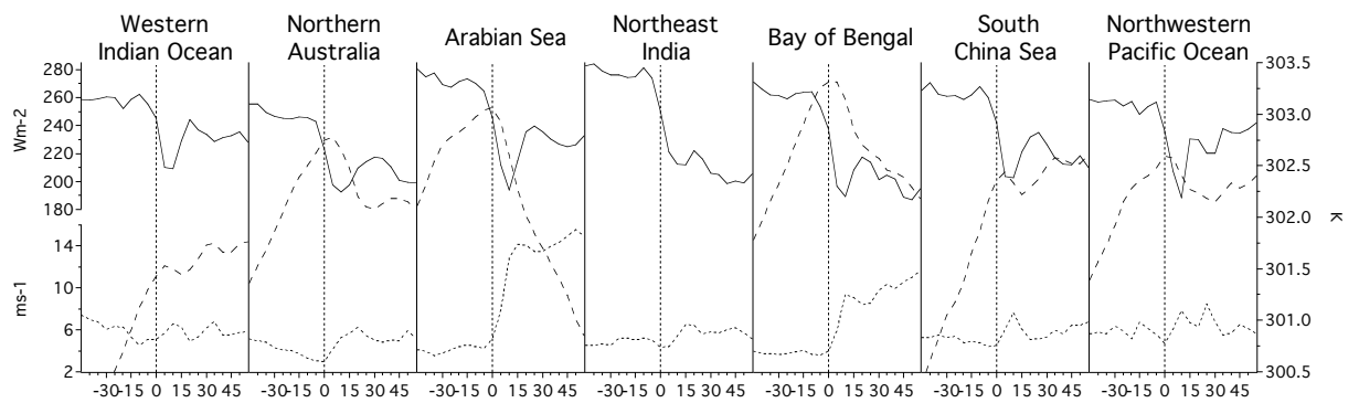
Figure 3.11 Composites des signaux régionaux moyennés sur 5 jours pour les forts évènements convectifs intrasaisonniers repérés à moins de 20 jours de la DMDP pour l'OLR (trait continu), la vitesse du vent à 850 hPa (pointillés) et la température de surface de l'océan (tirets). L'origine de l'abscisse est le moment de maximum de diminution de l'OLR.
