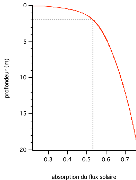
Figure 5.1 Fraction du flux solaire incident absorbée dans la couche mélangée océanique (Soloviev, 1982).
