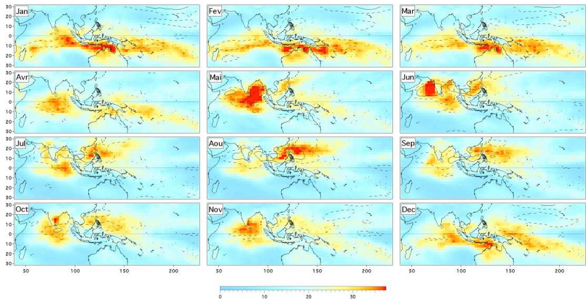
Figure 3.3 Ecart type moyen mensuel dans la bande 20-90 jours pour l'OLR ( Wm^{-2} , couleurs) et le vent à 850hPa NCEP (contour continu : 3,5 ms^{-1} ; tirets : 2,5 ms^{-1} ).
