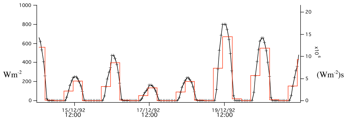
Figure 5.5 Cycles diurnes du flux solaire incident ( Wm^{-2} ) reconstruits d'après les données ERA 40 (4 fois par jour) au point 1^{\circ}45' S , 156^{\circ} N (zone IFA de TOGA COARE) et les intégrales sur 6 heures correspondantes données par ERA-40.
