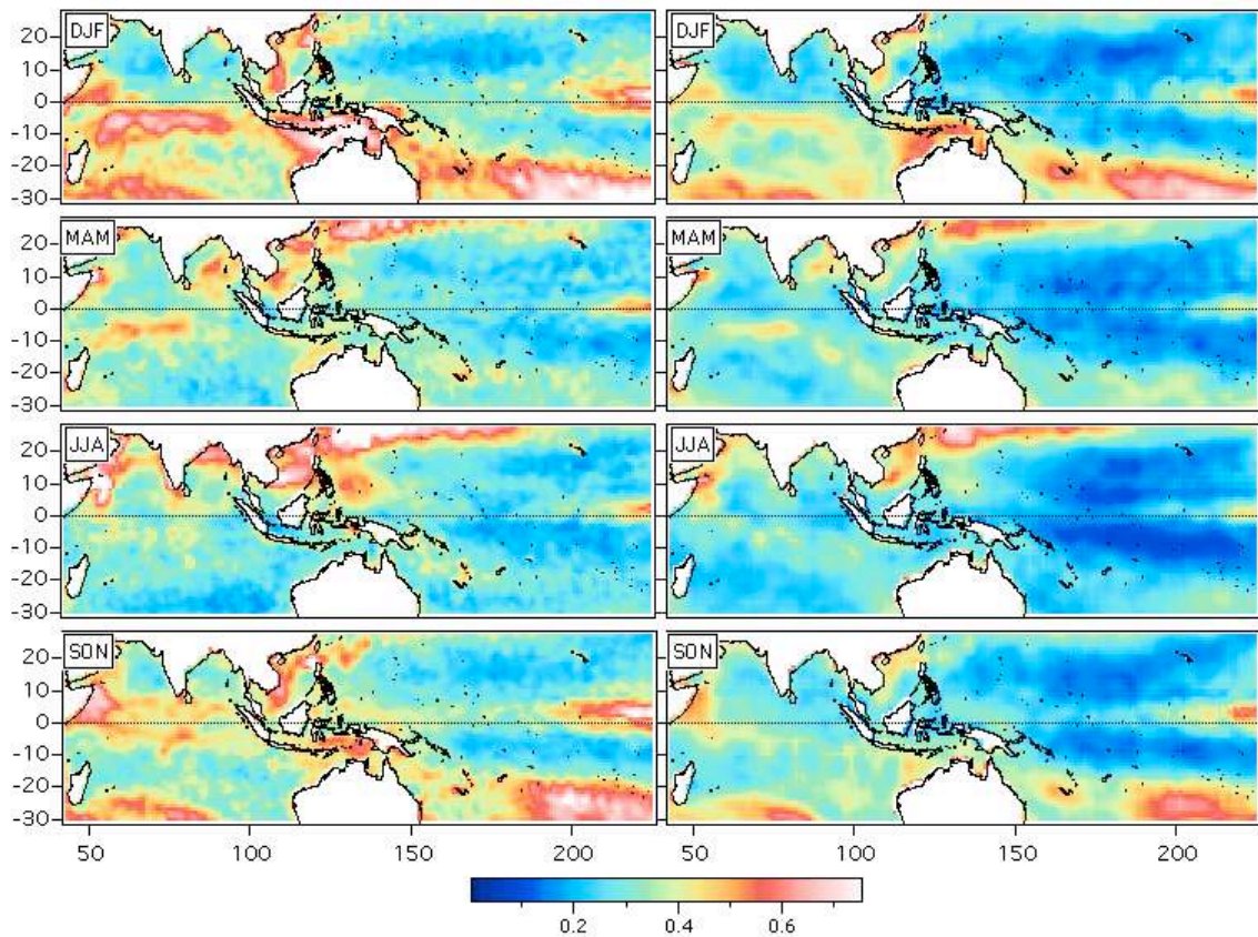
Figure 2.3 Distributions moyennes des écarts types de la TSO pour les variations de périodes 20-90 jours pour les années 1998-2004 (gauche) températures TMI, et (droite) températures Reynolds en °C.
