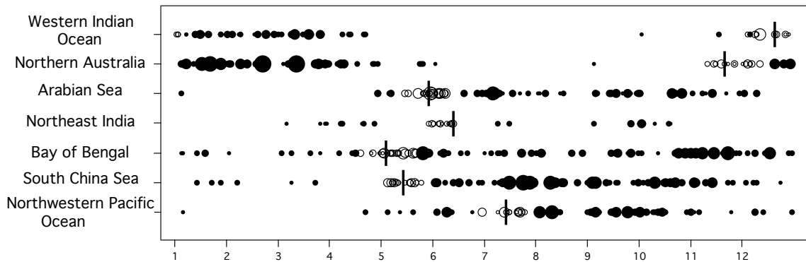
Figure 3.10 Distribution des plus forts évènements convectifs intrasaisonniers (cercles) avec un cercle vide pour ceux qui se situent à moins de 20 jours de la DMDP. La taille des cercles est proportionnelle à l'amplitude de l'événement (différence entre le maximum d'OLR filtré et le minimum suivant de 40 à 110 Wm^{-2} ). La DMDP est repérée pour chaque région par le trait vertical.
