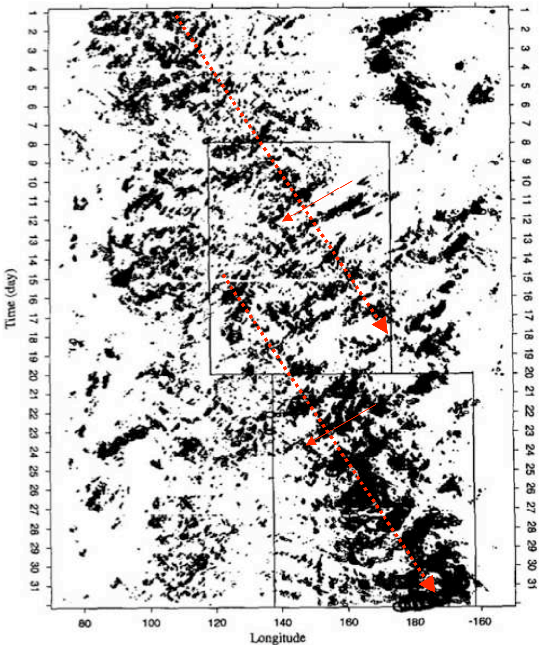
Figure 1.10 Diagramme temps-longitudes (moyenne sur 0°-10° sud) des amas convectifs (température de brillance <208K) pour le mois de décembre 1992. D'après Yanai et al (2000).
