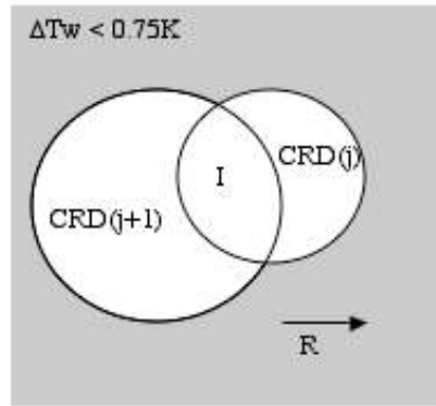
Figure 5.30. On définit une CRD très réactive comme étant la surface connexe définie par le contour \Delta T_w = 0.75K (variation diurne). Deux CRD de deux jours consécutifs ( j et j+1 ) font partie d'une même CRDP si R est suffisamment grand ( > 875 Km) et que l'intersection I entre elle soit au moins un tiers de la superficie de la plus petite des deux CRD. Une CRDP est constituée d'au moins 5 CRD consécutives remplissant ces conditions.
