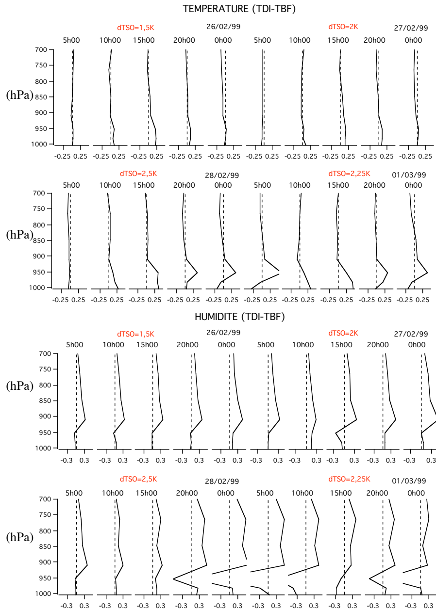
Figure 6.13 Profils des différences de température ( ^{\circ}\text{C} ) et d'humidité ( \text{g/kg} ) entre TDI et TBF pour la région 63^{\circ}\text{E } 8^{\circ}\text{S} . Les variations diurnes de TSO pour chaque jour sont rappelés ( d\text{TTSO} en rouge).
