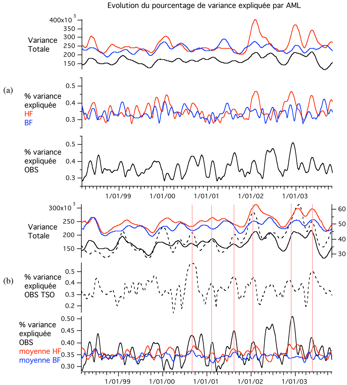
Figure 4.13 (a) Evolutions temporelles de la variance (20-60 jours) totale sur la région d'étude (30°-180°E, 30°S-30°N) et du Pourcentage de Variance Expliquée (PVE) par l'AML pour l'OLR observé, et l'OLR d'un membre de chacun des ensembles de simulations. (b) comme (a) mais la variance totale et PVE du modèle sont les moyennes pour chaque ensemble, la variance totale et le PVE de la TSO sont reportés en pointillés.
