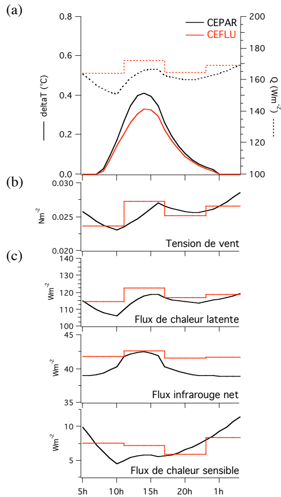
Figure 5.6 Evolutions quotidiennes composites pour les méthodes CEPAR (noir) et CEFLU (rouge) pour novembre-décembre 1992 au point 2.5^{\circ}\text{S} , 156^{\circ}\text{E} (zone IFA de TOGA COARE). (a) Variation diurne de la température de surface de l'océan due à une CRD (trait continu, K) et pertes totale d'énergie Q à la surface (pointillés, \text{Wm}^{-2} ). (b) tension du vent à la surface ( \text{Nm}^{-2} ). (c) flux de chaleur latente (trait continu gras), flux de chaleur sensible (trait continu fin) et flux infrarouge net (pointillés) en \text{Wm}^{-2} .
