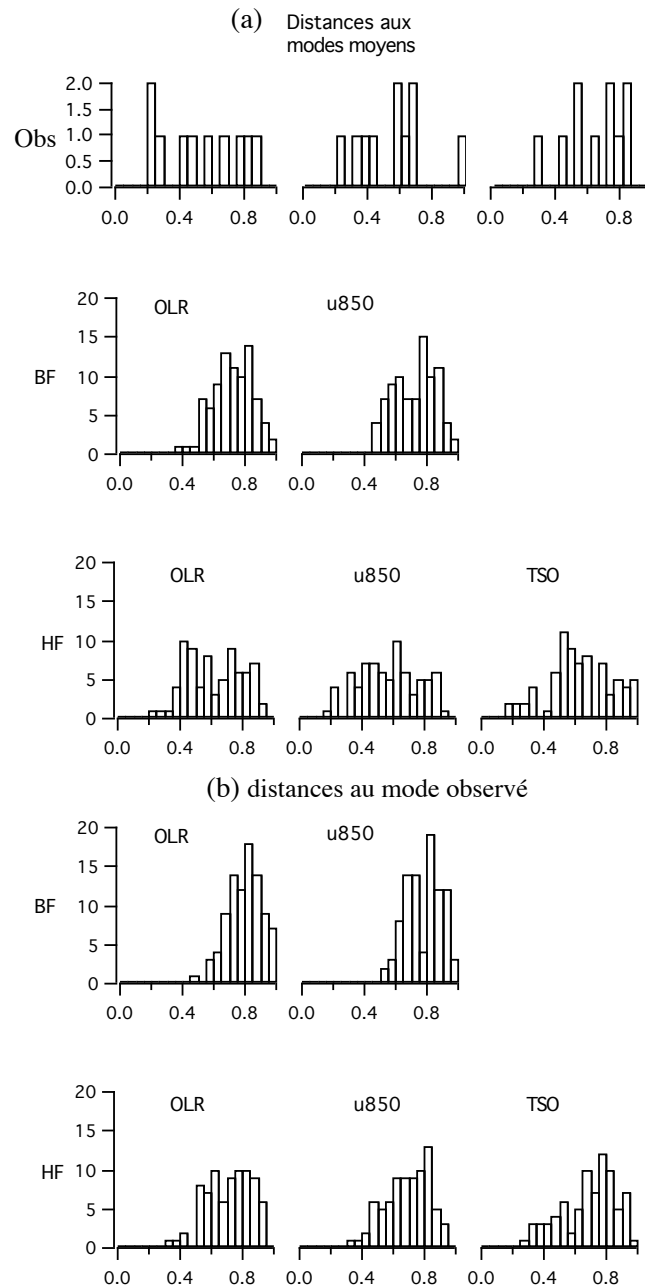
Figure 4.16 (a) Distribution des distances aux événements intrasaisonniers moyens d'hiver respectifs pour les observations (et réanalyses) et les ensembles BF et HF des événements intrasaisonniers d'hiver. (b) Distances à l'événement moyen hivernal observé des événements des ensembles BF et HF.
