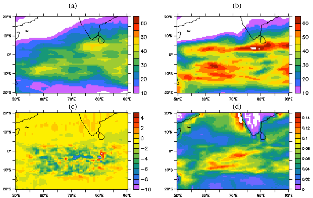
Figure 13. Variabilité 10-45 jours pour les trois premiers mois de 1999 de (a) l’OLR NOAA ( Wm^{-2} ), (b) OLR simulation TBF ( Wm^{-2} ), et les différences entre les variabilités 10-45 jours des simulations TDI et TBF pour les trois premiers mois de 1999 de (c) l’OLR ( Wm^{-2} ), (d) la température de surface océanique ( ^{\circ}C ).
