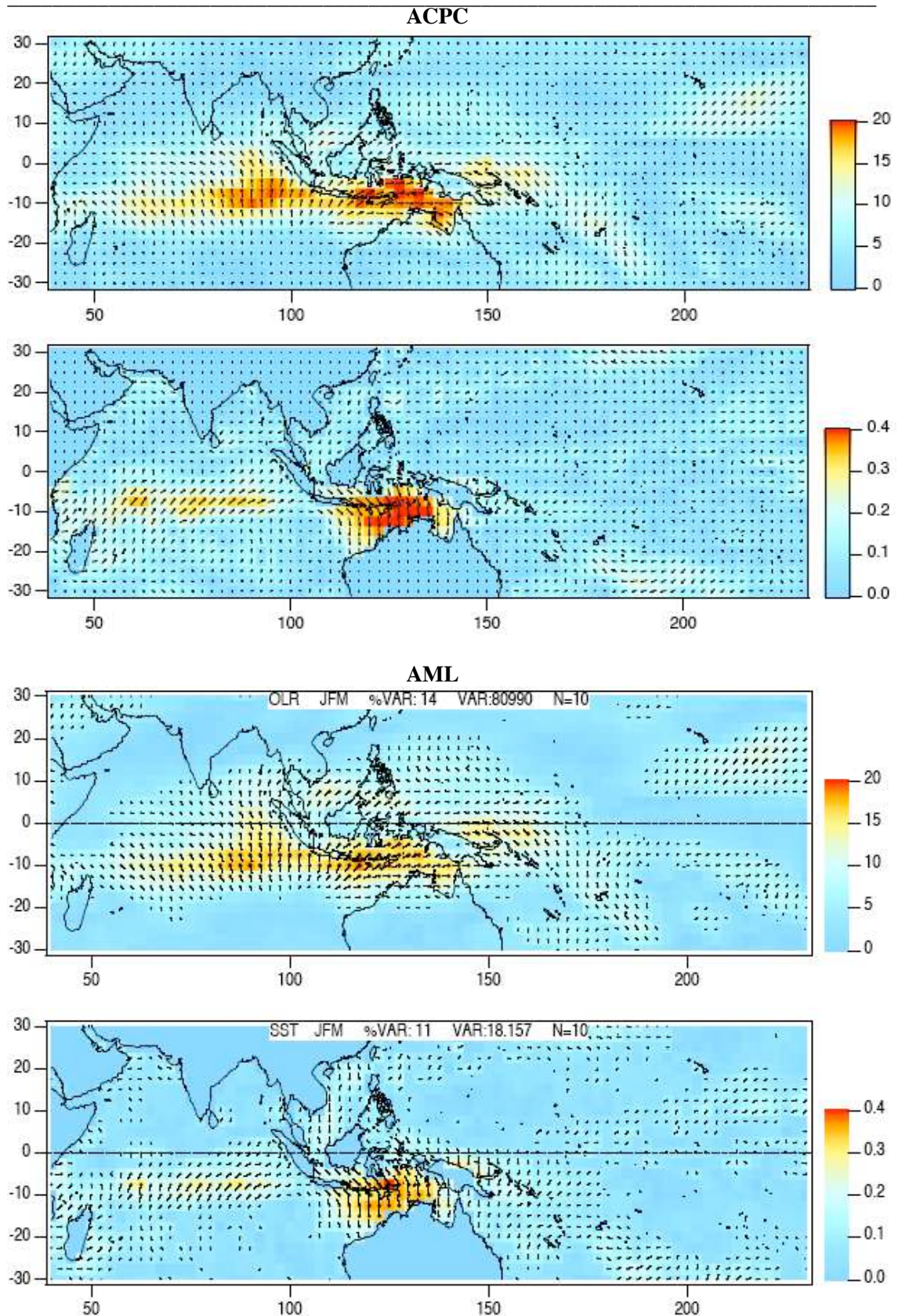
Figure 2.15 Structures spatiales des modes moyens d'OLR ( Wm^{-2} ) et de TSO ( ^{\circ}C ) sur la période 1998-2004 pour (haut) l'ACPC sur 7 fenêtres de 90 jours et (bas) l'AML sur 10 fenêtres de 120 jours.
