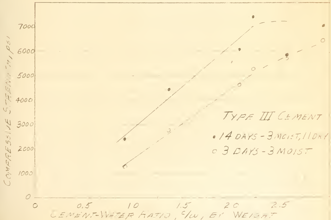
FIG. E12 - TRIAL BATCHES
