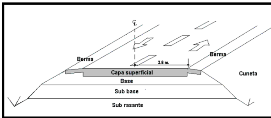
Figura 4: Espesores del pavimento flexible
