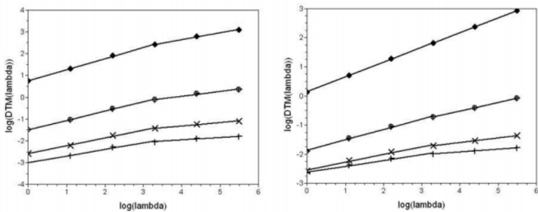
Figure 10 : DTM ( q=1.5 , \eta=0.66 ; 1 ; 1.52 ; 2.31 ) en fonction de la résolution en graphique log-log pour l'analyse spatio-temporelle en moyenne d'ensemble. (à gauche) Simulation Més0-NH (à droite) Données radar. Les coefficients de régression linéaire R^2 pour les grandes échelles, pour les petites échelles et sans prendre en compte de rupture valent respectivement 0.99, 0.98 et 0.97 pour les données Més0-NH et 0.99, 0.99 et 0.98 pour les données radar.
