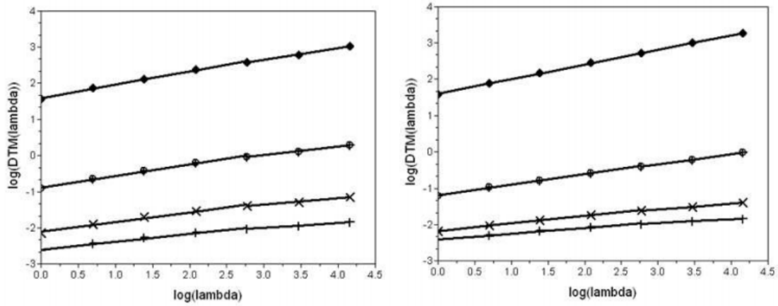
Figure 7 : DTM ( q=1.5 , \eta=0.66 ; 1 ; 1.52 ; 2.31) en fonction de la résolution en graphique log-log pour l'analyse temporelle en moyenne d'ensemble. (à gauche) Simulation Més0-NH (à droite) Données radar. Les coefficients de régression linéaire R^2 pour les grandes échelles, pour les petites échelles et sans prendre en compte de rupture valent respectivement 0.99, 0.99 et 0.98 pour les données Més0-NH et 0.99, 0.99 et 0.99 pour les données radar.
