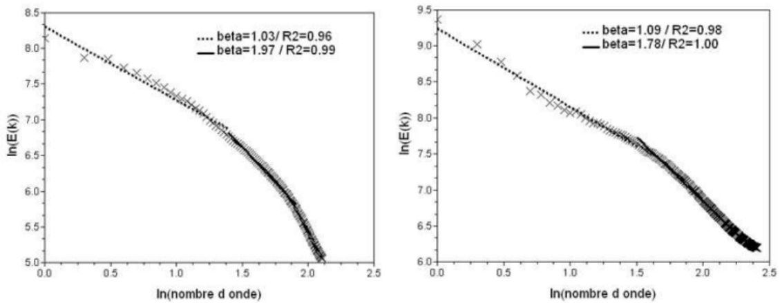
Figure 2 : Moyenne d'ensemble des spectres en analyse spatiale : Méso-NH (à droite) et radar (à gauche)
