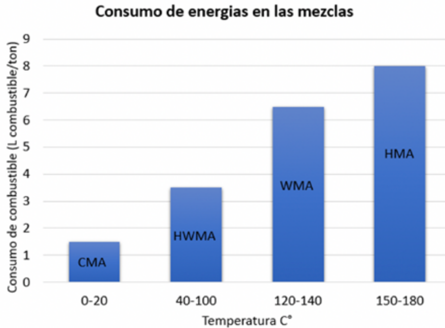
Figura 1. Clasificación de las mezclas asfálticas de acuerdo con la temperatura. Fuente: Elaboración propia, modificado de [5].
