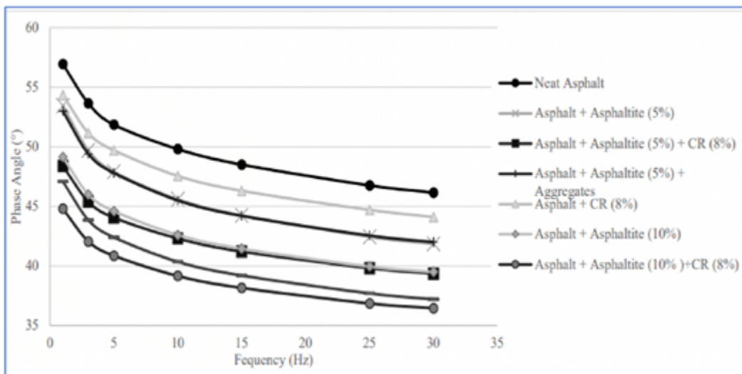
Figura 4. Ángulo de fase a 22 °C para todas las muestras modificadas con HMA. Fuente: Tomado de [25].
