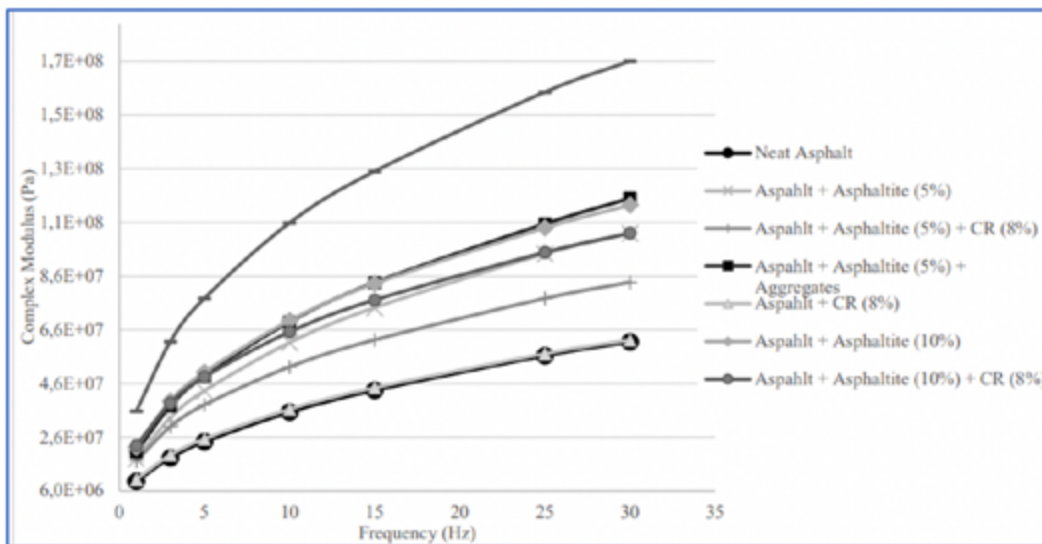
Figura 3. Módulo dinámico a 22 °C para todas las muestras modificadas con HMA. Fuente: Tomado de [25].
