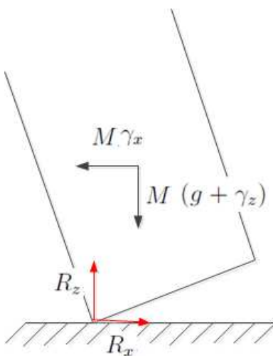
FIGURE 3.1 – Schéma d'un cube basculant
