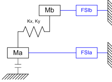
FIGURE 4.2 – Schéma du modèle Masses-Ressort
