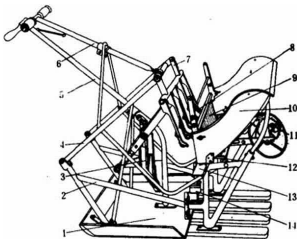
图8 借鉴了莳耜工作原理的人力梳式插秧机
