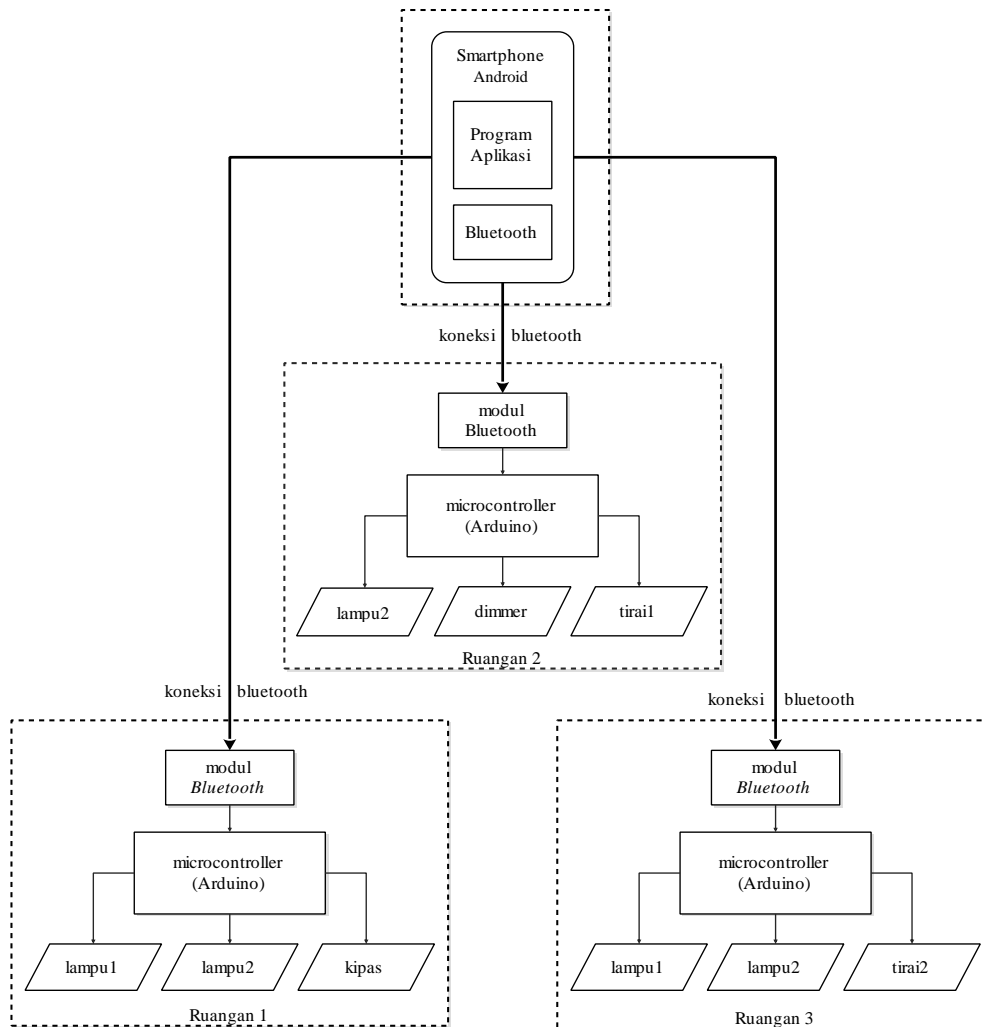
Gambar 1 Arsitektur sistem
