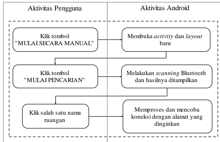
Gambar 3 Detail proses pencarian secara maual
