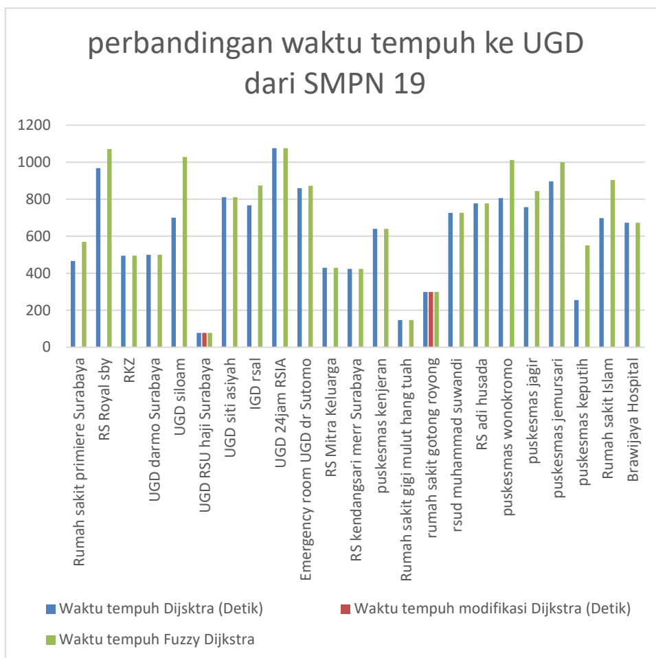
Gambar 3. Grafik perbandingan waktu tempuh ke UGD dari SMPN 19 dari ketiga algoritma pukul 09:00-09:10 WIB.
