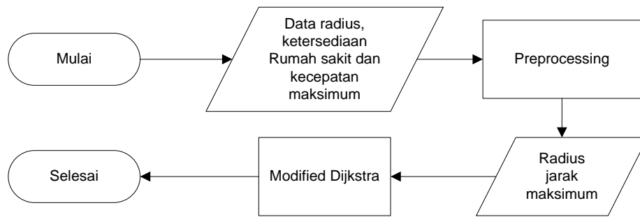
Gambar 1. Digram alir metode modifikasi Dijkstra.
