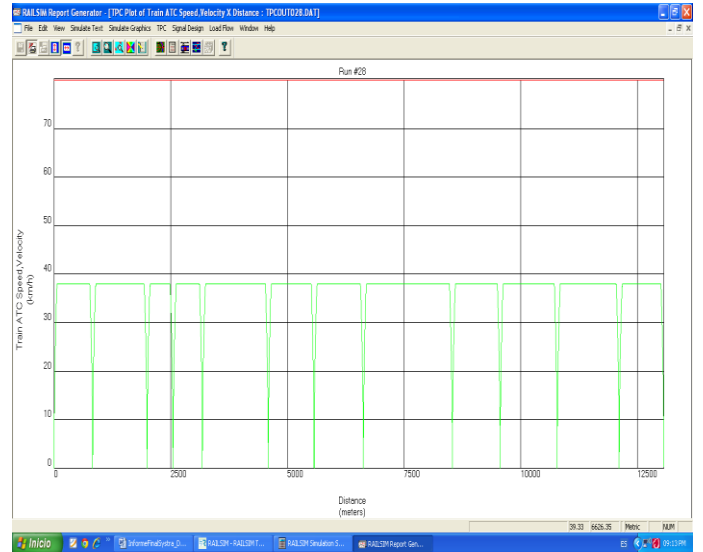
Figura 8. Run#28, régimen de velocidad de 38 km/h.
