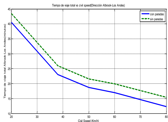
Fig 6. Tiempo total vs. Velocidad máxima (civil speed).
