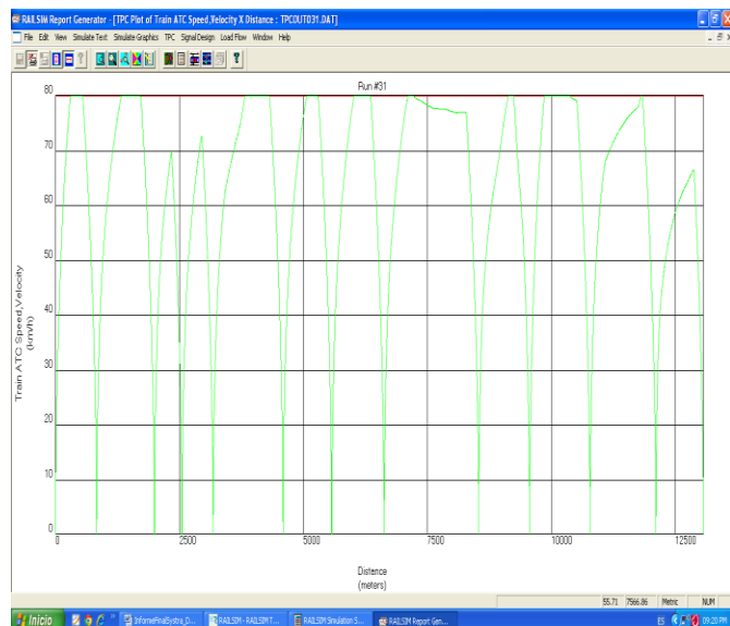
Figura 10. Run#15, régimen de velocidad de 80 km/h
