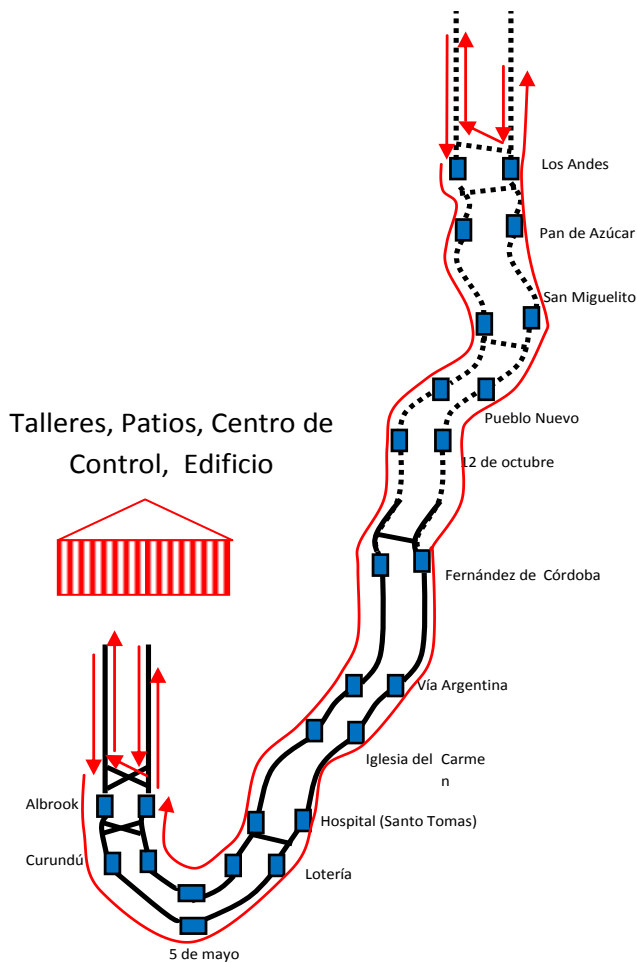
Figura.5. Esquema del movimiento de trenes durante los servicios nominales Fuente: A. Berbey-Alvarez. Project characterization of Panama metro rail system. Facultad de Ingeniería Eléctrica. Universidad Tecnológica de Panamá.
