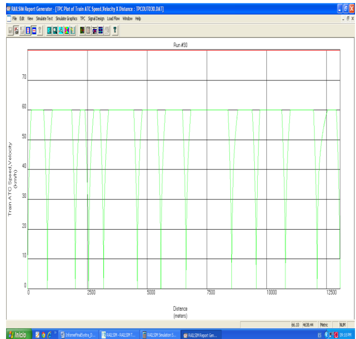
Figura 9. Run#30, régimen de velocidad de 60 km/h.
