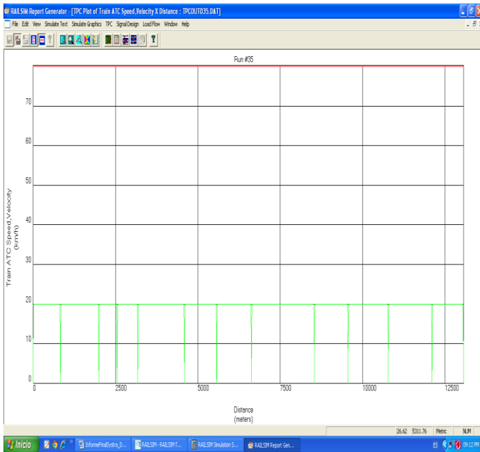
Figura 7. Run#35, régimen de velocidad límite 20km/h.
