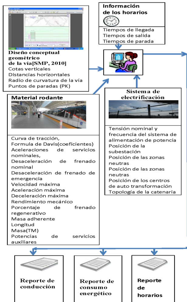
Figura 4. Esquema general para la realización de simulaciones ferroviarias de la línea 1 del metro de Panamá. Fuente: A. Berbey-Alvarez. Project characterization of Panama metro rail system. Facultad de Ingeniería Eléctrica. Universidad Tecnológica de Panamá.
