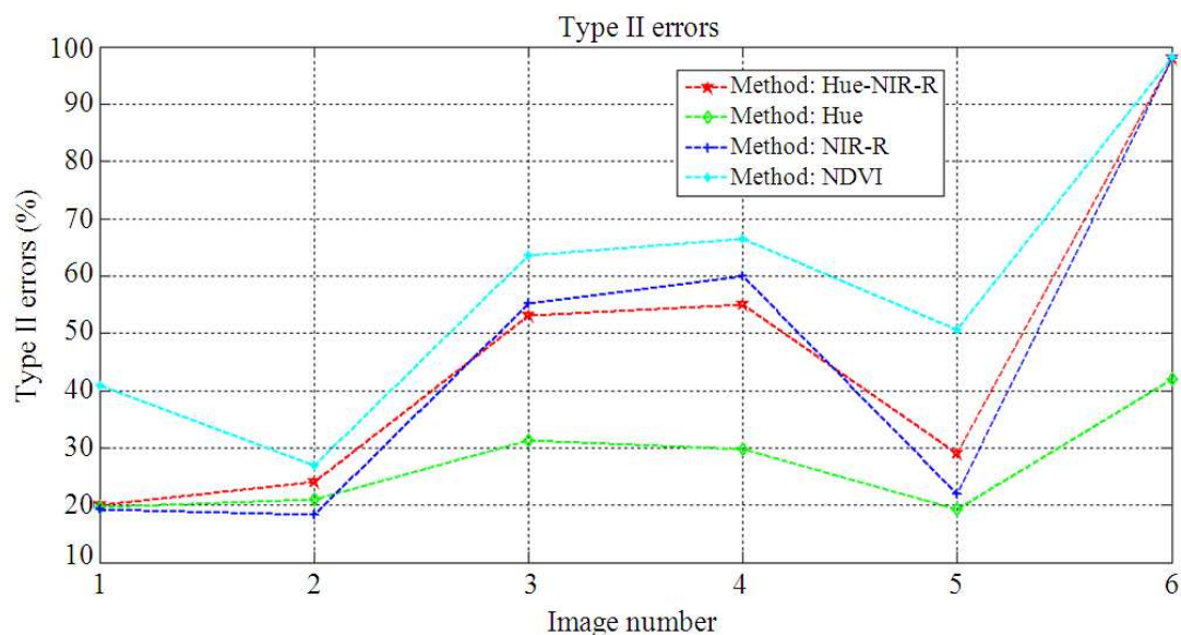
Fig. 10. Type II error
