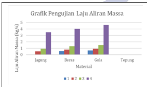
Gambar 12. Grafik Rata-rata Nilai Laju Aliran Massa
