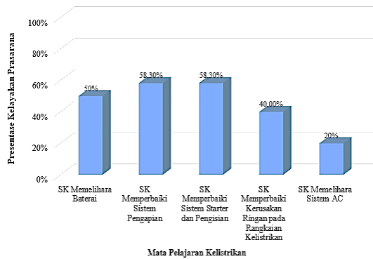
Gambar 1. Persentase Pencapaian Standar Prasarana Praktik Kelistrikan Program Keahlian Teknik Kendaraan Ringan SMK Negeri 1 Kalitengah
