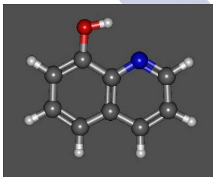
Gambar 1. Pemodelan Senyawa 8-Hidroksiquinolin Dasar Menggunakan Software Gabedit 2.4.0
