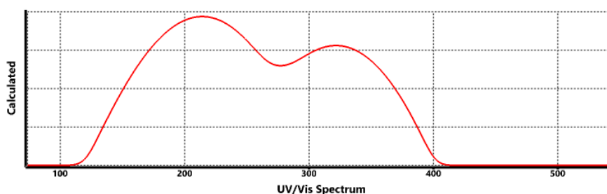
Gambar 8. Spektra UV-Vis 8-hidroksiquinolin dasar
