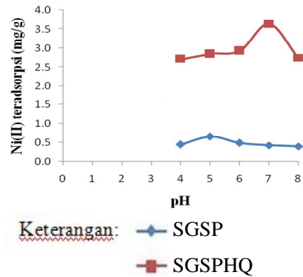
Gambar 4. Adsorpsi Ni(II) pada berbagai pH medium oleh Silika gel Sekam Padi dan Hibrida Silika Gel Sekam Padi Hidroksiquinolin (SGSPHQ)
