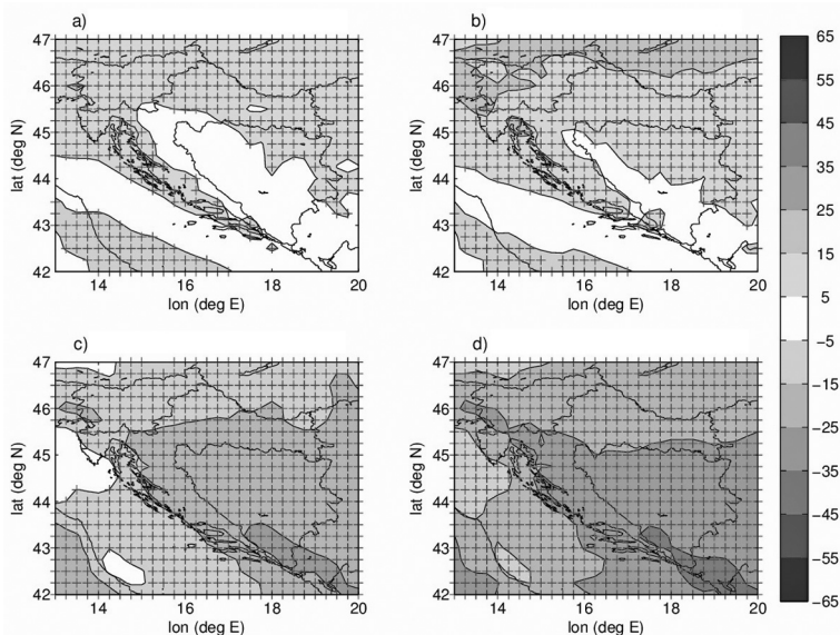
Slika 9. Promjena ukupne oborine (u %) u odnosu na referentno razdoblje 1961.–1990. za zimu (gore) i ljeto (dolje) za razdoblje 2041.–2070. (lijevo) i razdoblje 2071.–2100. (desno). S oznakom + označene su točke u kojima dvije trećine modela daje isti predznak promjene kao srednjak skupa klimatskih modela.
