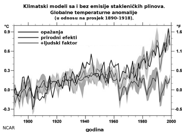
Slika 5. Simulacija opažene promjene temperature u 20. stoljeću. (Izvor: www.met.ed.ucar.edu ).
