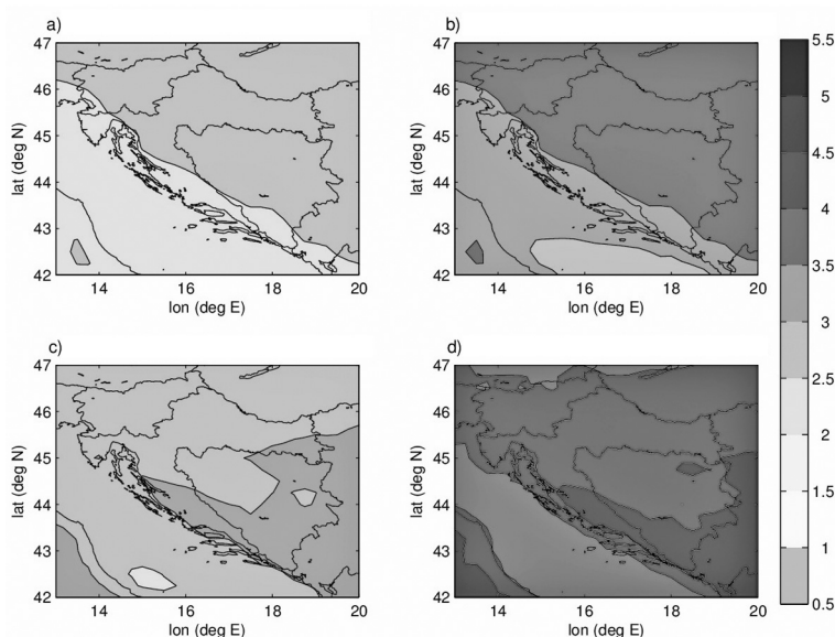
Slika 8. Promjena temperature na 2 m (u °C) u odnosu na referentno razdoblje 1961.–1990. za zimu (gore) i ljeto (dolje) za razdoblje 2041.–2070. (lijevo) i razdoblje 2071.–2100. (desno). U svim točkama dvije trećine modela daje isti predznak promjene kao srednjak skupa klimatskih modela.
