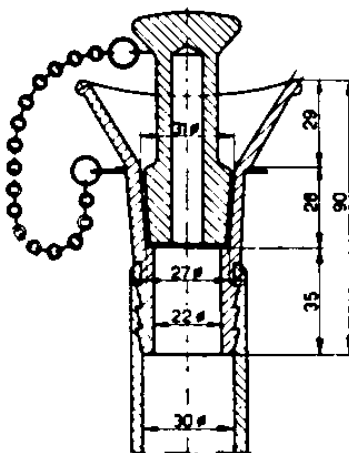
Sl. 1 Izgled brodskog dojavnog zvukovoda
