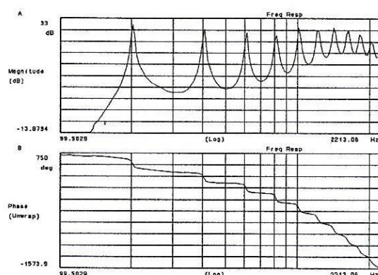
Sl. 3 Izmjerena amplitudna i fazna frekvencijska karakteristika l = 0.81 \text{ m} 2r = 0.041 \text{ m}
