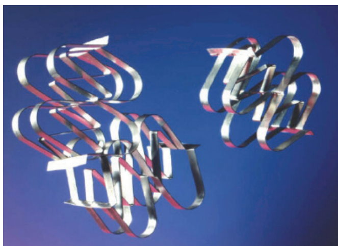
Slika 4 – Raschigovi superprsteni
